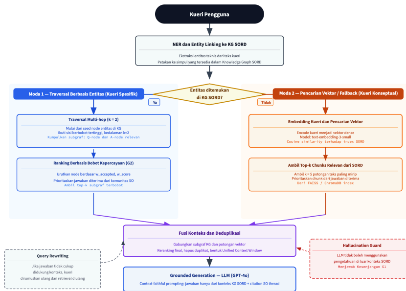
Gambar III.5 Flowchart alur pemrosesan kueri pada GraphRAG Framework .
