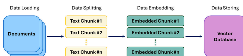
Gambar II.4 Proses pengindeksan pada pipeline RAG: mulai dari pemuatan data ( data loading ), pemotongan teks ( chunking ), pembentukan embedding, hingga penyimpanan dalam basis data vektor ( vector database ). (Kamalipour2026)
