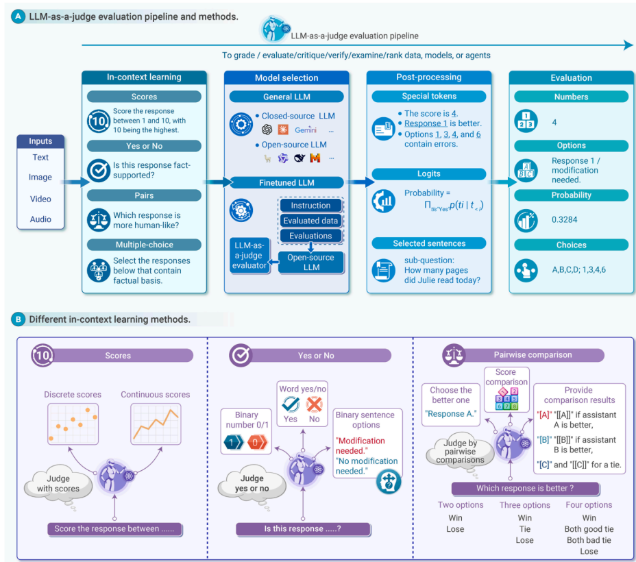
Gambar II.9 (A) Pipeline evaluasi LLM-as-a-judge dari awal hingga akhir, mencakup empat tahap. (B) Metode penilaian: scoring , classification , dan ranking . Gu, Jiang, Shi, dkk. (2026)
