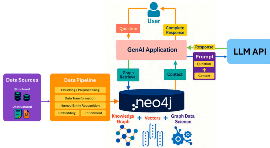
Gambar II.6 Gambaran umum pipeline Graph-RAG: ekstraksi triple, penelusuran subgraf ( sub-graph traversal ), serta integrasi hibrida antara representasi vektor dan simbolik.(Kamalipour, Asadi, dan Chimeh 2026)
