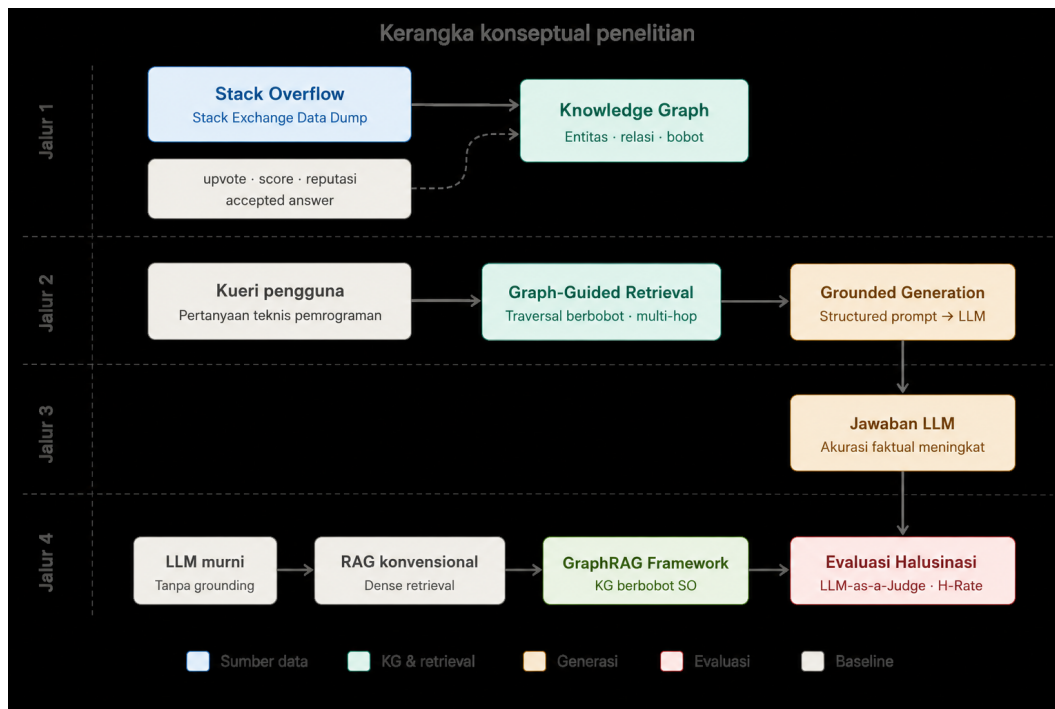
Gambar II.10 Kerangka konseptual penelitian: integrasi Stack Overflow sebagai sumber pengetahuan tervalidasi sosial, knowledge graph berbobot sebagai struktur representasi, mekanisme graph-guided retrieval , grounded generation , dan protokol evaluasi halusinasi.
