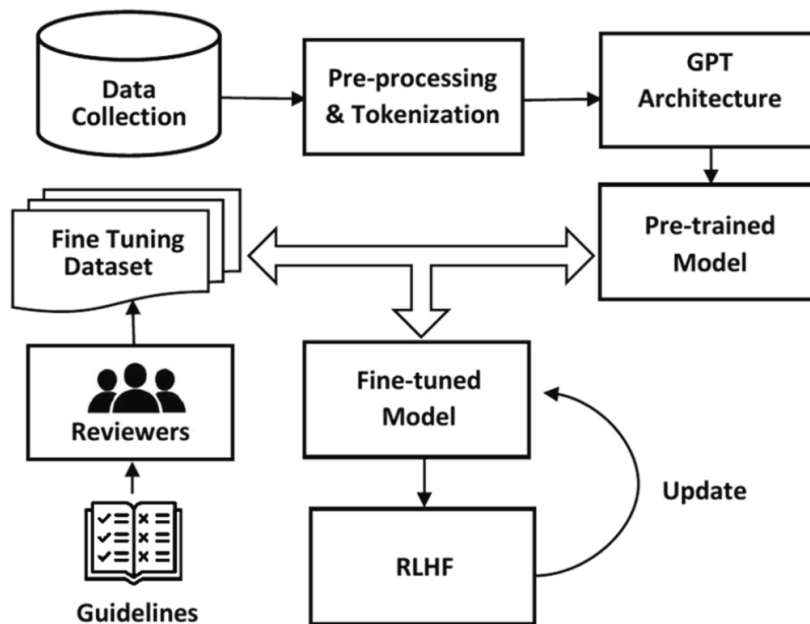
Gambar II.2 Tahapan pelatihan ChatGPT yang meliputi pre-training , supervised fine-tuning , dan RLHF Haque (2025)
