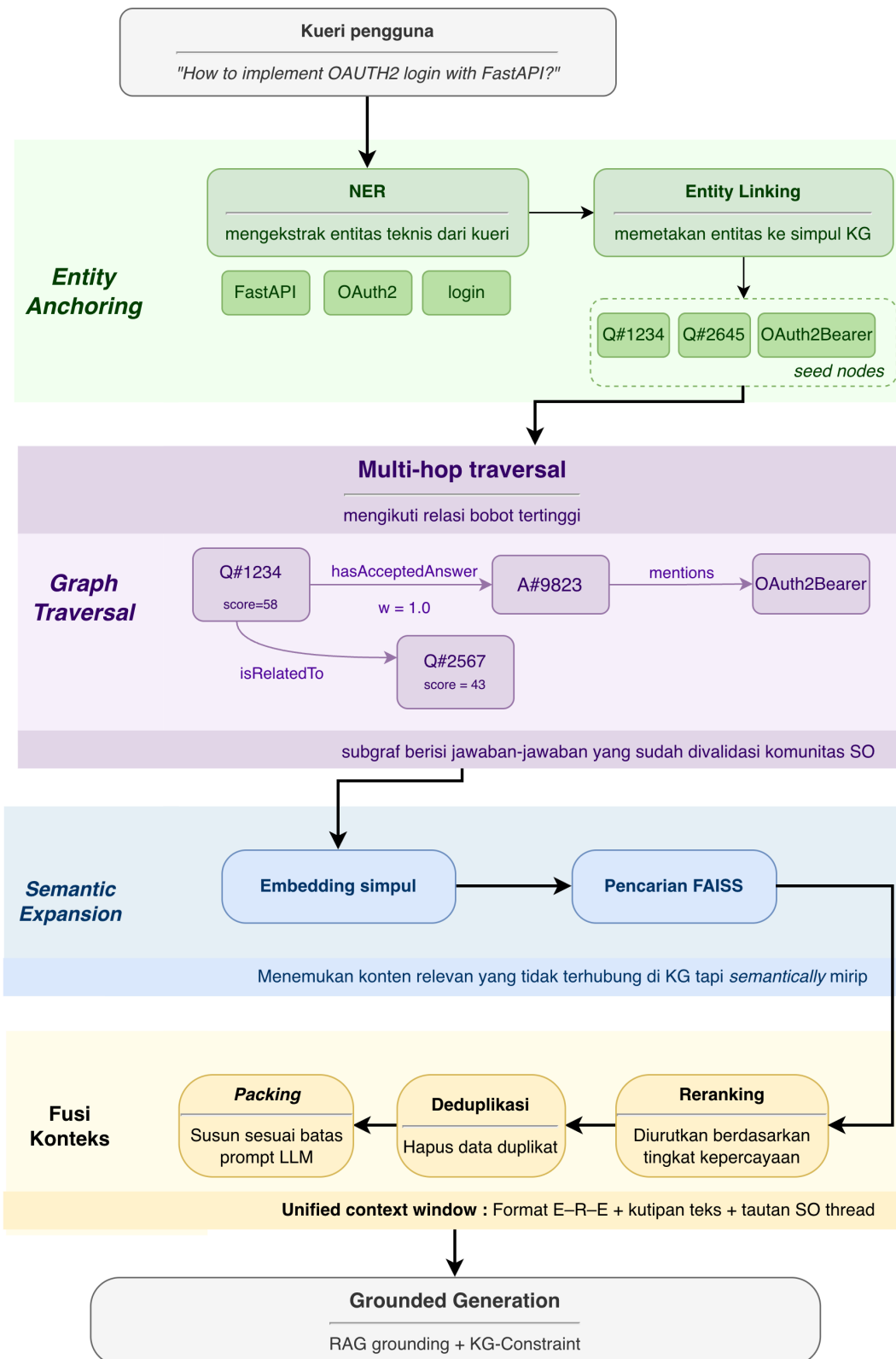
Gambar III.6 Alur mekanisme hybrid retrieval pada GraphRAG Framework .
