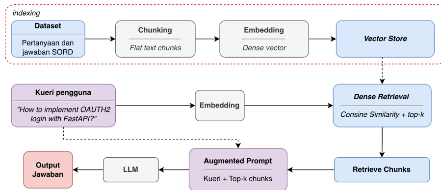
Gambar III.2 Arsitektur RAG Konvensional, diadaptasi dari taksonomi empat tahap (Kamalipour, Asadi, dan Chimeh 2026)
