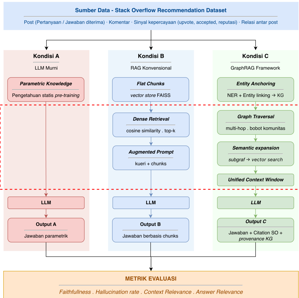
Gambar III.7 Perbandingan tiga kondisi evaluasi yang menghasilkan output yang diukur dengan metrik yang identik.
