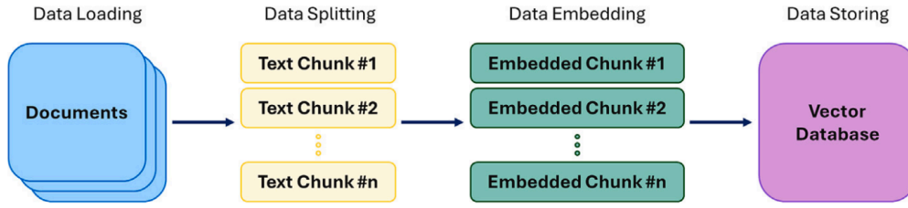
Gambar II.4 Proses pengindeksan pada pipeline RAG (Kamalipour, Asadi, dan Chimeh 2026).
