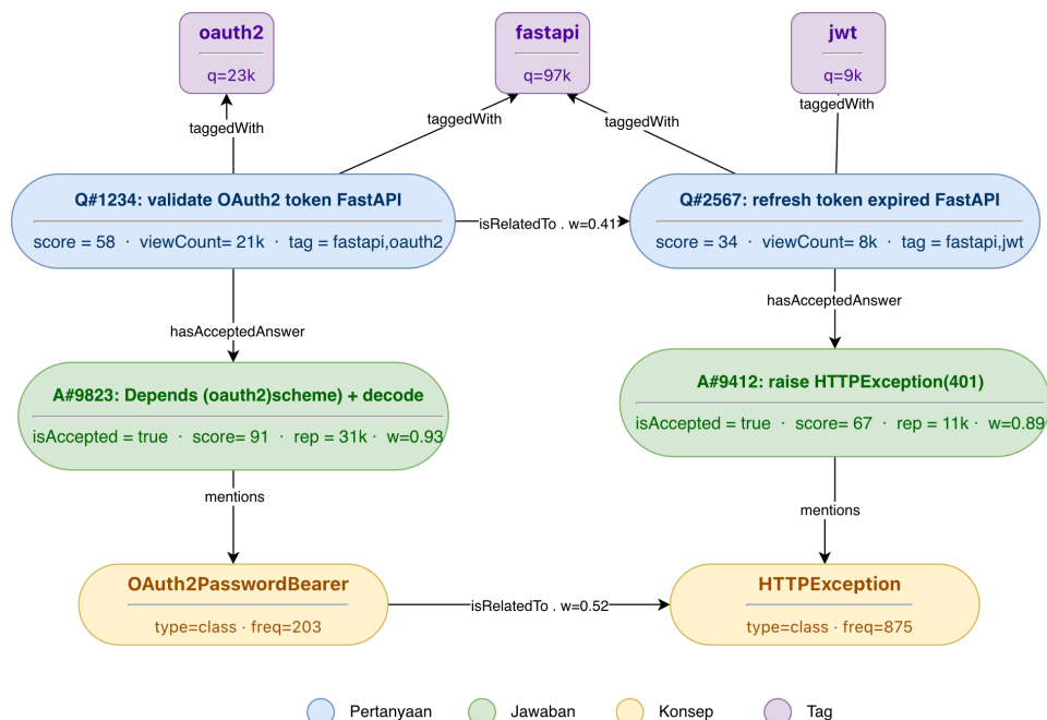
Gambar III.4 Contoh subgraf knowledge graph berbobot dari SORD pada domain autentikasi FastAPI
