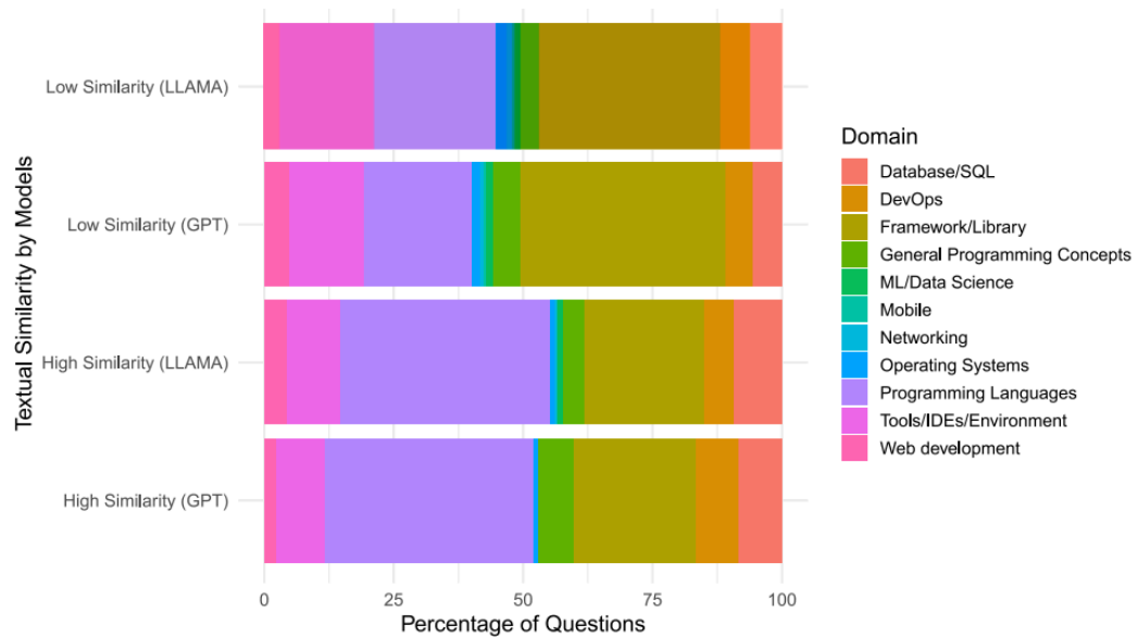
Gambar II.7 Distribusi domain pertanyaan untuk jawaban LLM dengan kemiripan tinggi dan rendah terhadap komunitas Stack Overflow. (Silva, Samhi, dan Khomh 2025)
