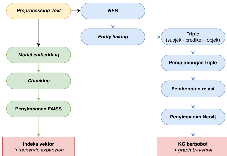
Gambar III.4 Flowchart konstruksi knowledge graph berbobot dari dataset SORD.
