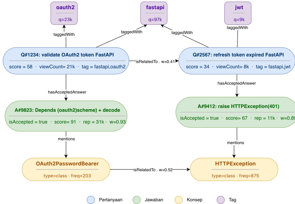
Gambar III.3 Contoh subgraf knowledge graph berbobot dari SORD pada domain autentikasi FastAPI
