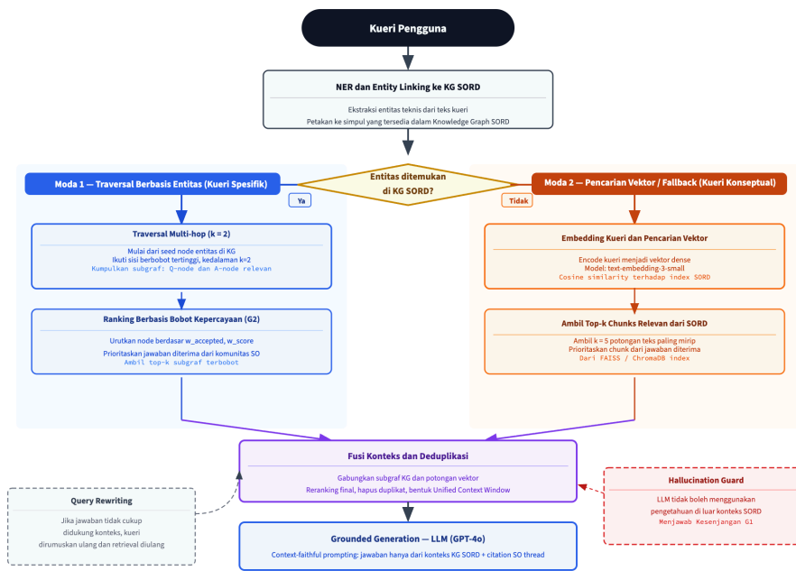
Gambar III.5 Flowchart alur pemrosesan kueri pada GraphRAG Framework .
