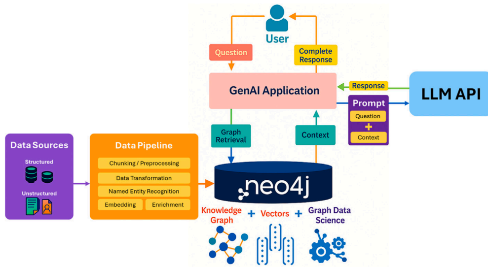
Gambar II.5 Gambaran umum pipeline Graph-RAG: ekstraksi triple, penelusuran subgraf ( sub-graph traversal ), serta integrasi hibrida antara representasi vektor dan simbolik. (Kamalipour, Asadi, dan Chimeh 2026)
