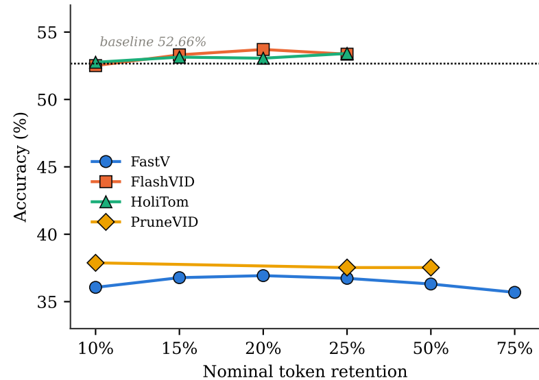
LLaVA-OV-7B
