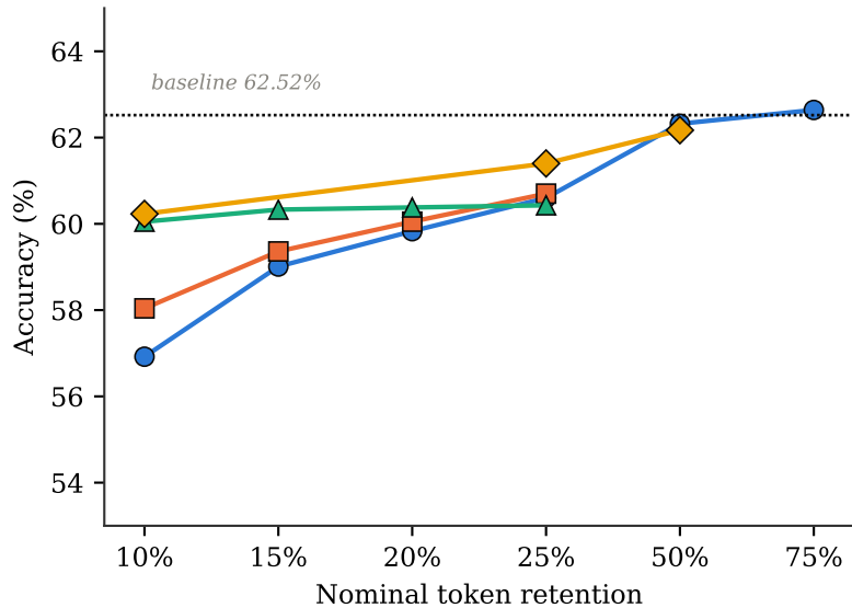
Qwen3-VL-8B
