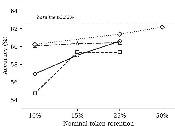
Qwen3-VL-8B
