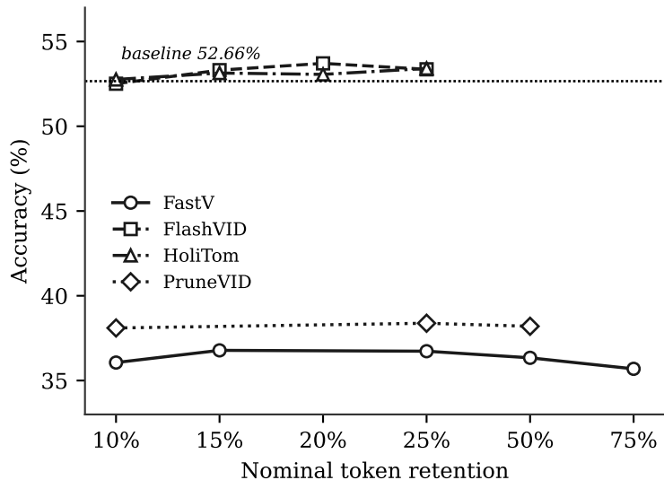
LLaVA-OV-7B
