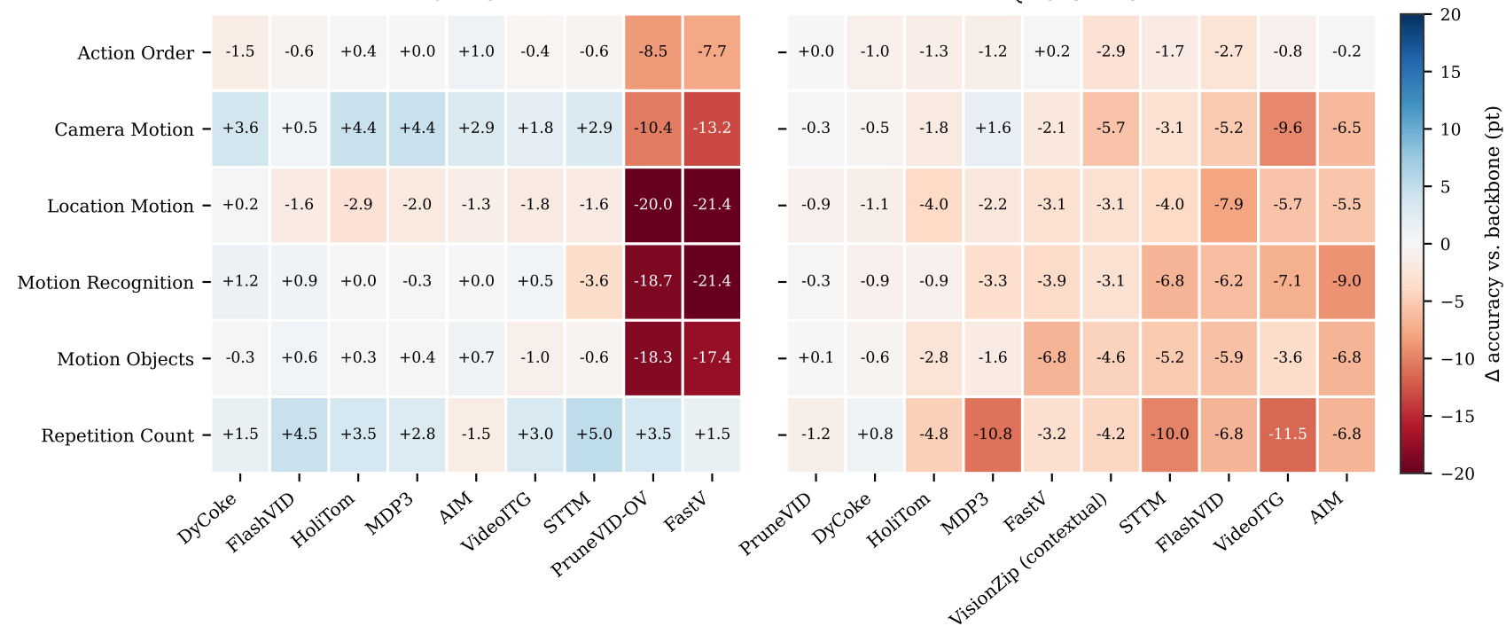
LLaVA-OV-7B
