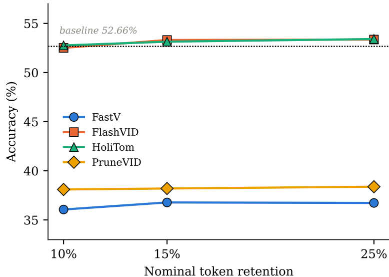
LLaVA-OV-7B
