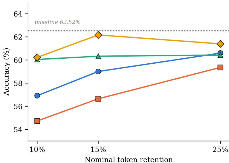
Qwen3-VL-8B
