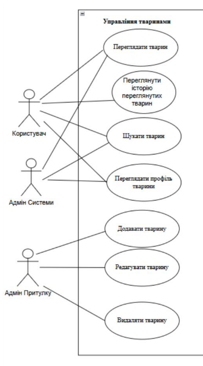
Рис. 5: Usecase - діаграма: Підсистема управління тваринами
