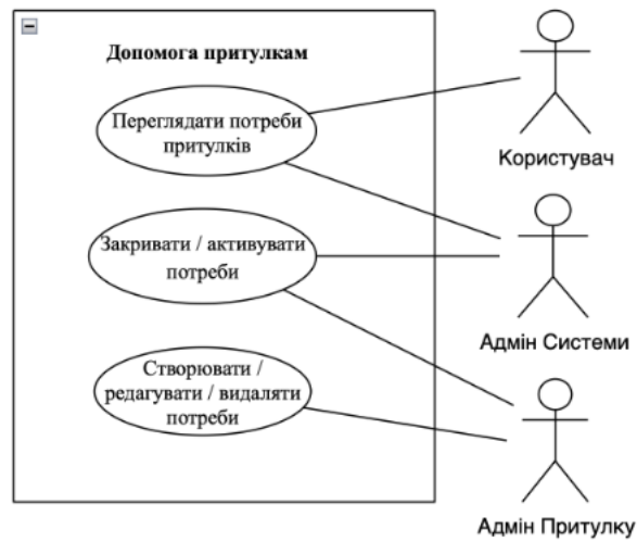
Рис. 3: Usecase - діаграма: Підсистема допомоги притулкам
