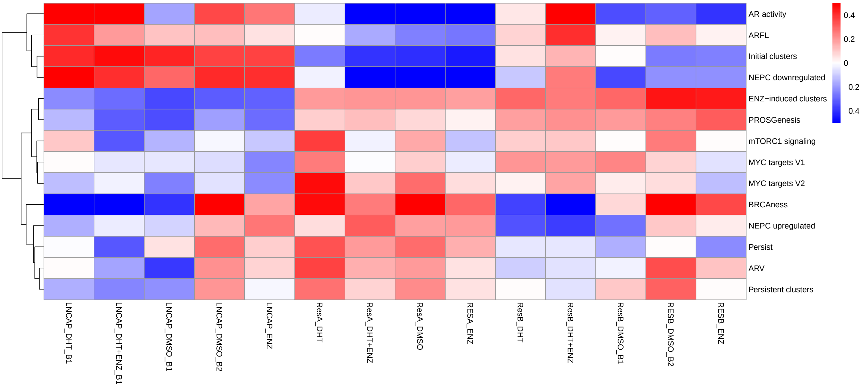
GSVA Plot Bulk RNA-seq
