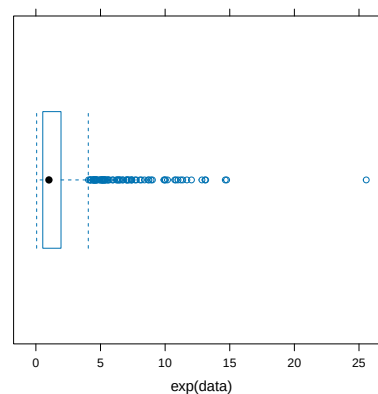
(d) Boxplot
