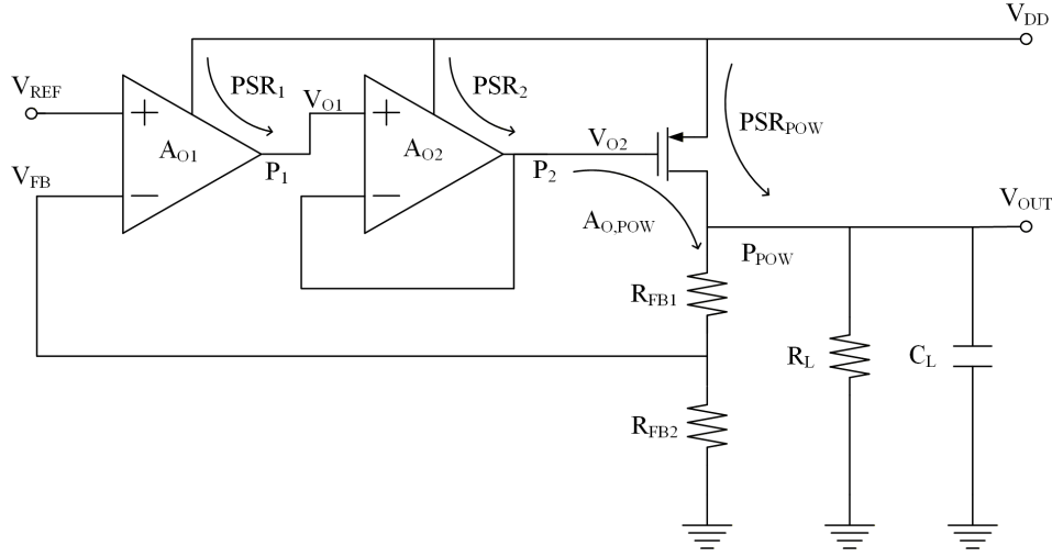
Figure 9 PSRR 分析示意图
