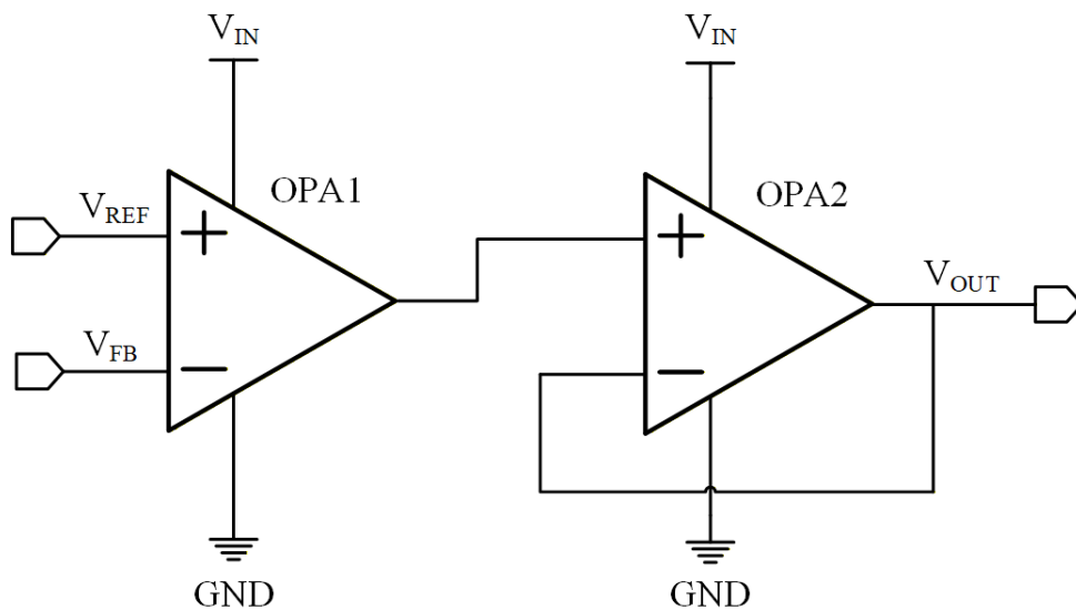
Figure 3 ea 架构示意图
