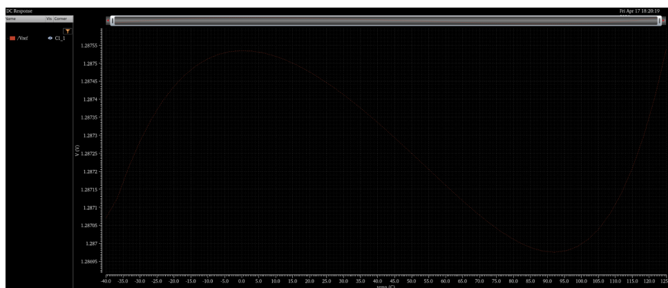
Figure 13 bandgap 在 tt 工艺角下的输出电压随温度变化的仿真结果
