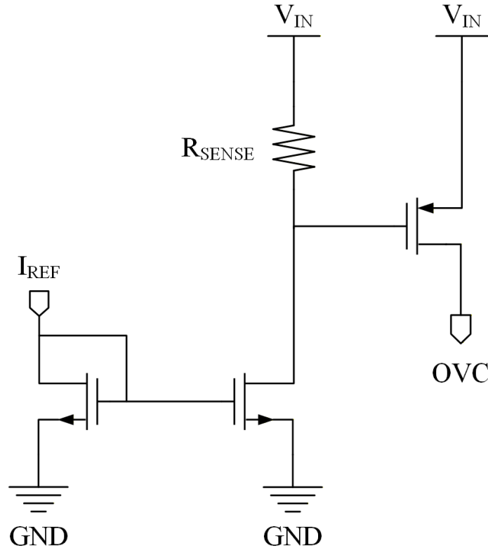
Figure 7 限流模块示意图
