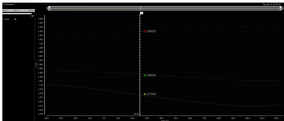
Figure 14 bandgap 调整电阻网络参数后的输出电压随温度变化的仿真结果
