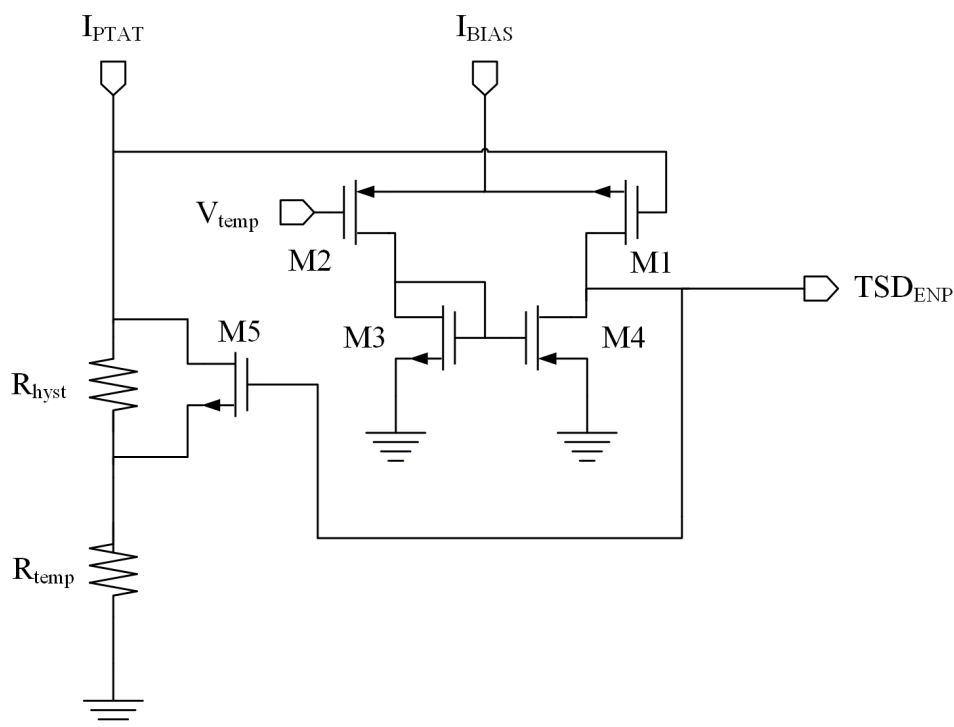
Figure 8 过温保护模块示意图
