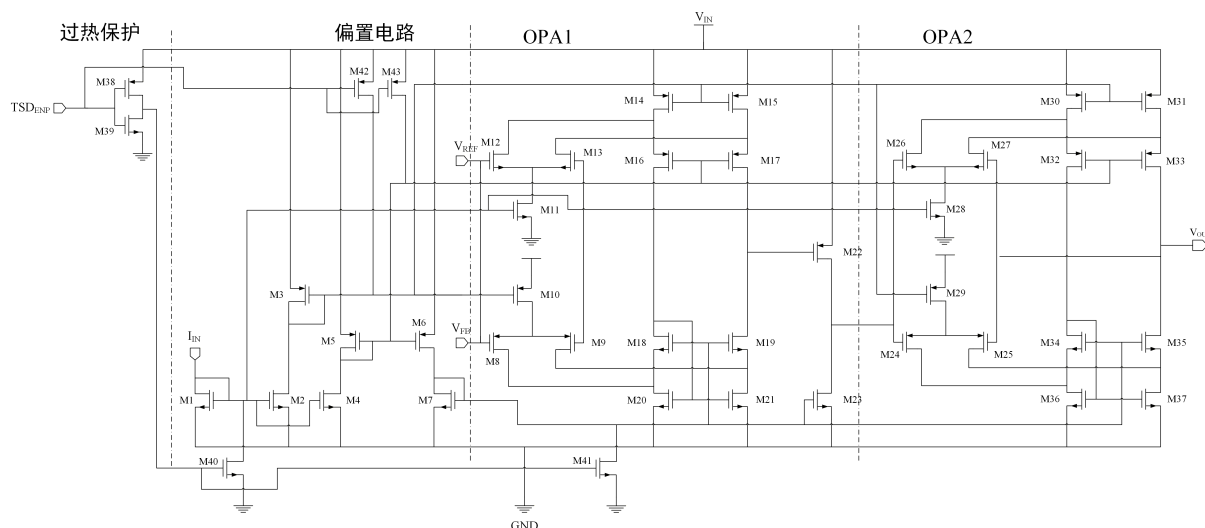
Figure 4 ea 详细电路图
