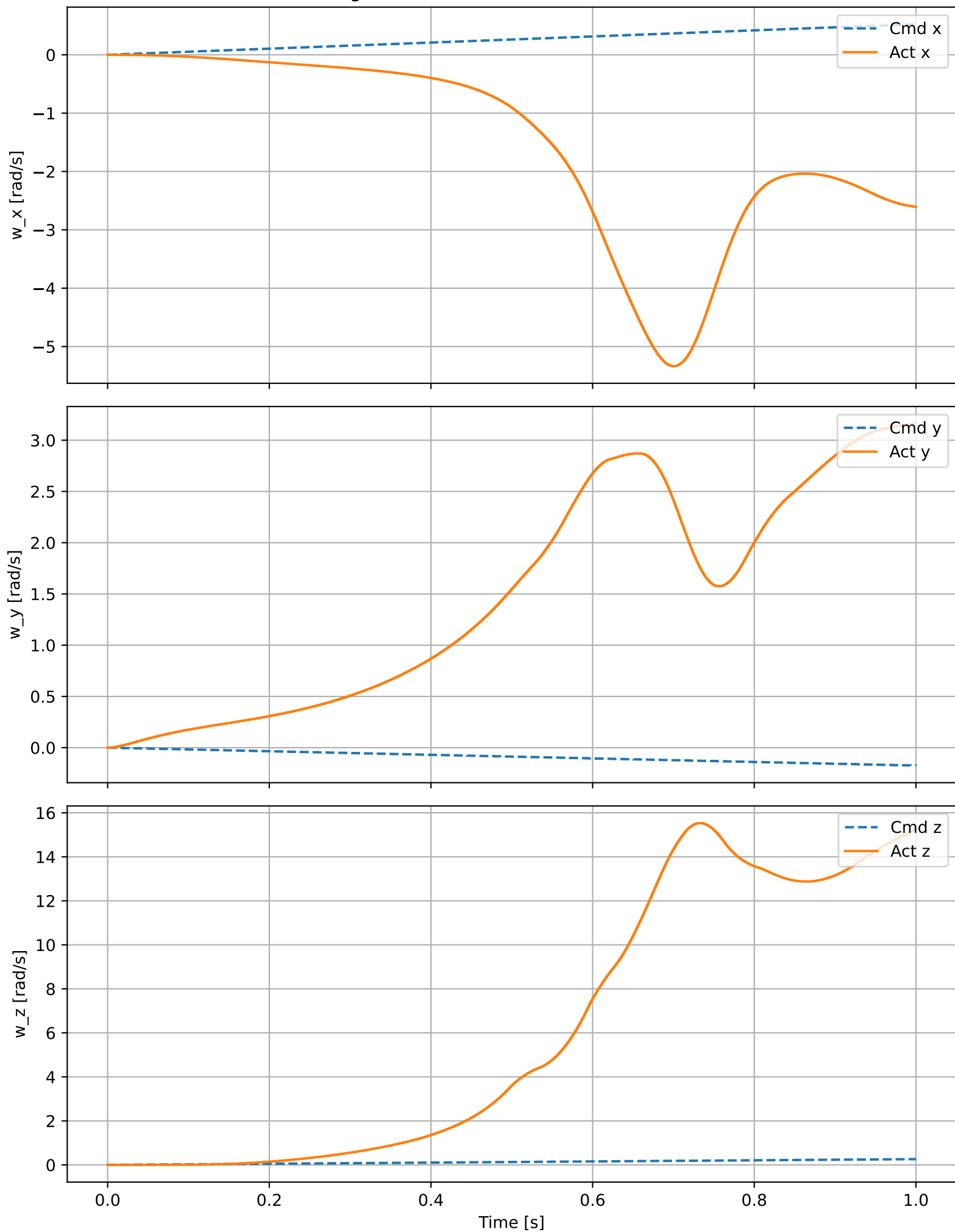
Angular Rates: Commanded vs. Actual
