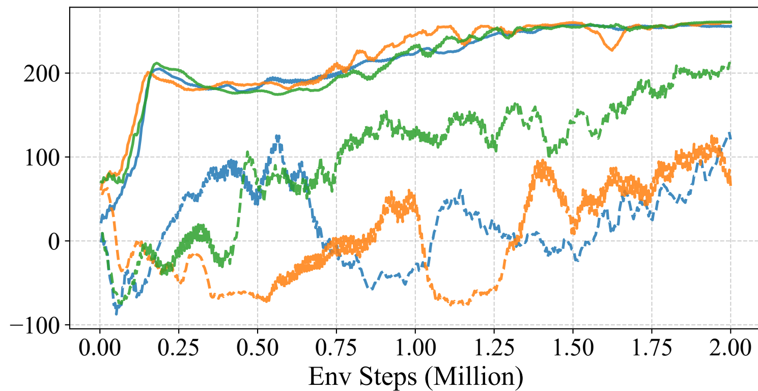
Eval Return
