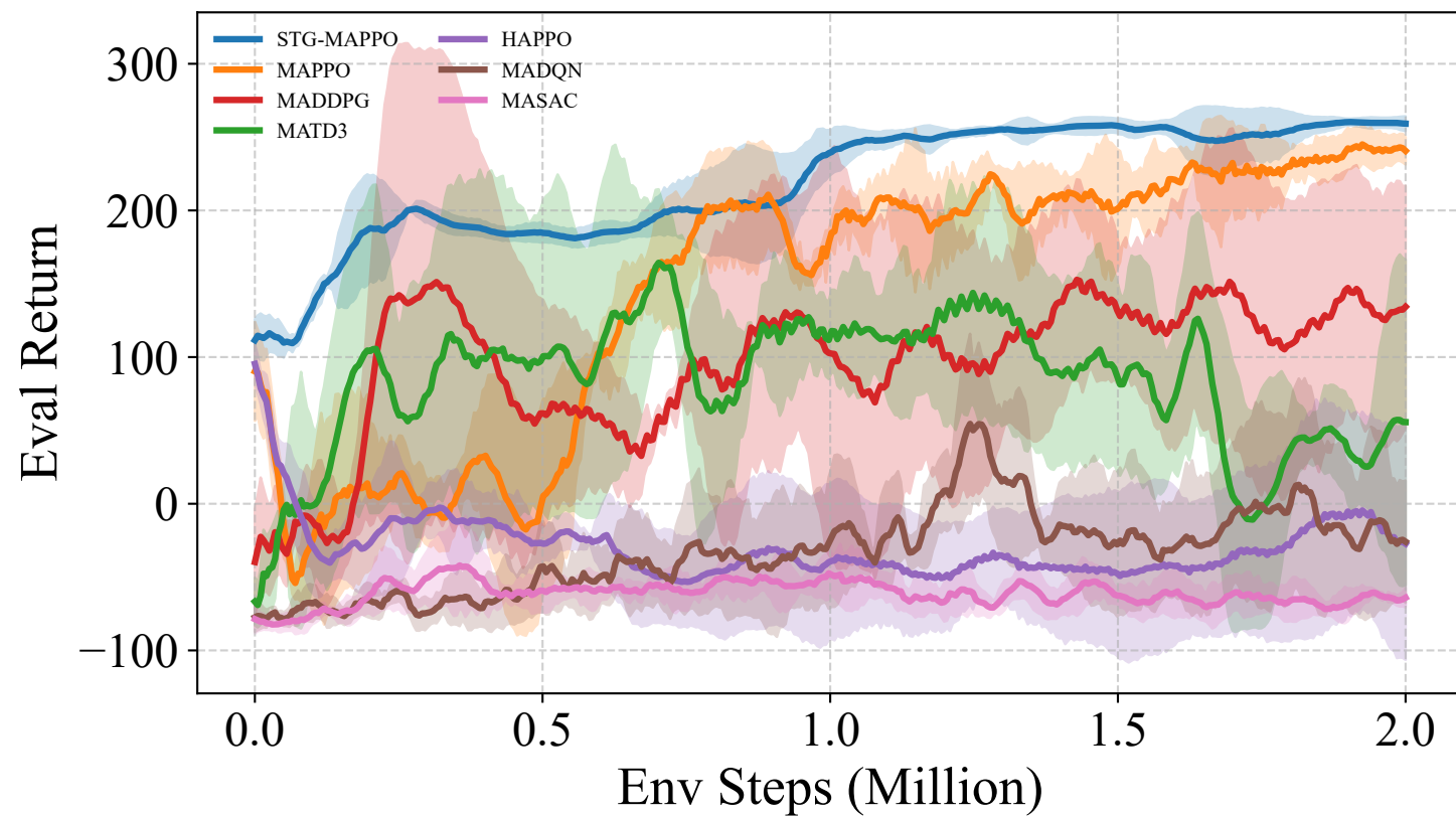
Eval Return
