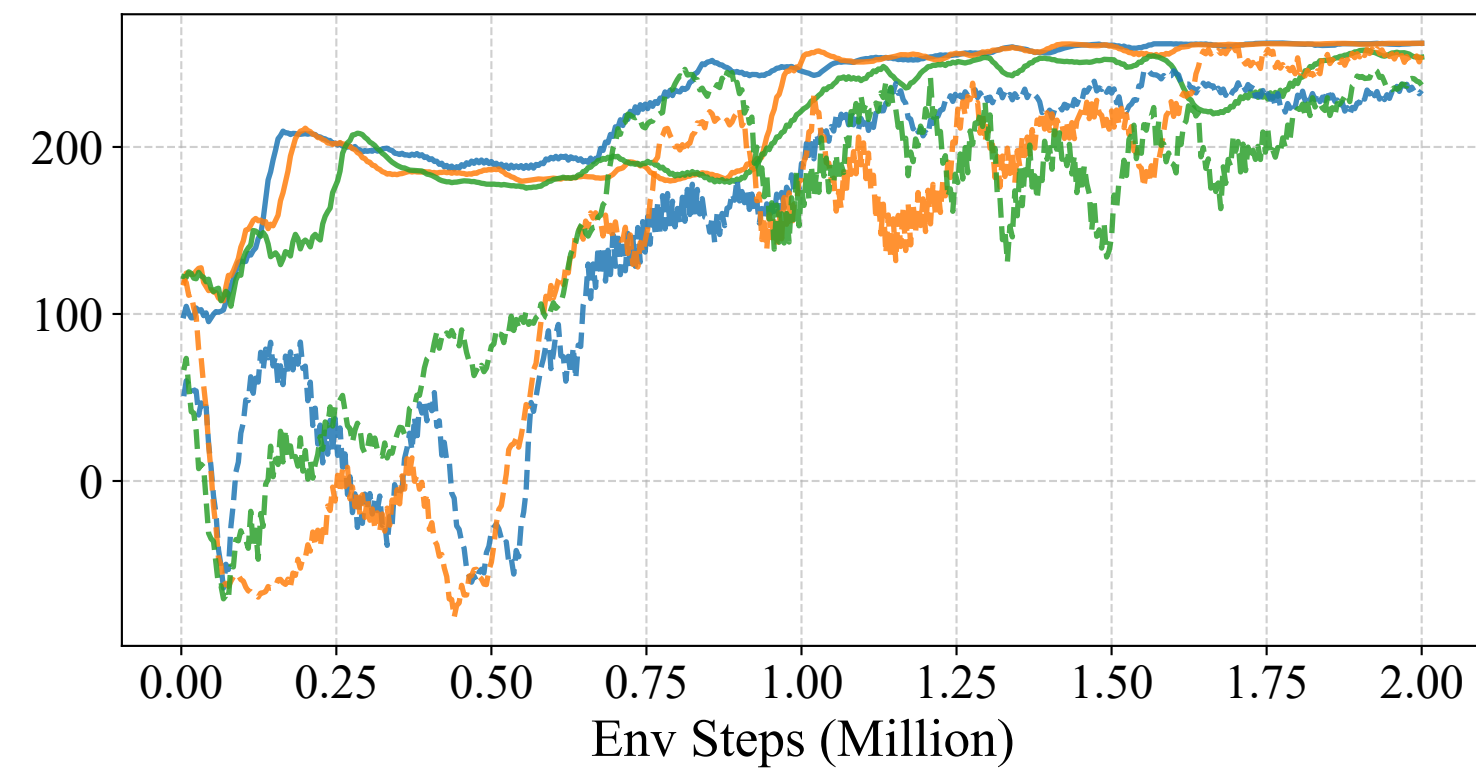
Eval Return
