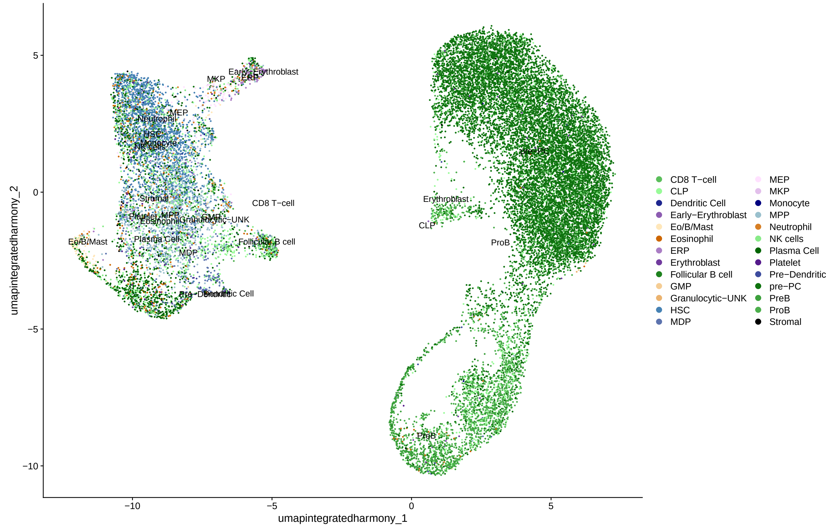
pred_celltypist
