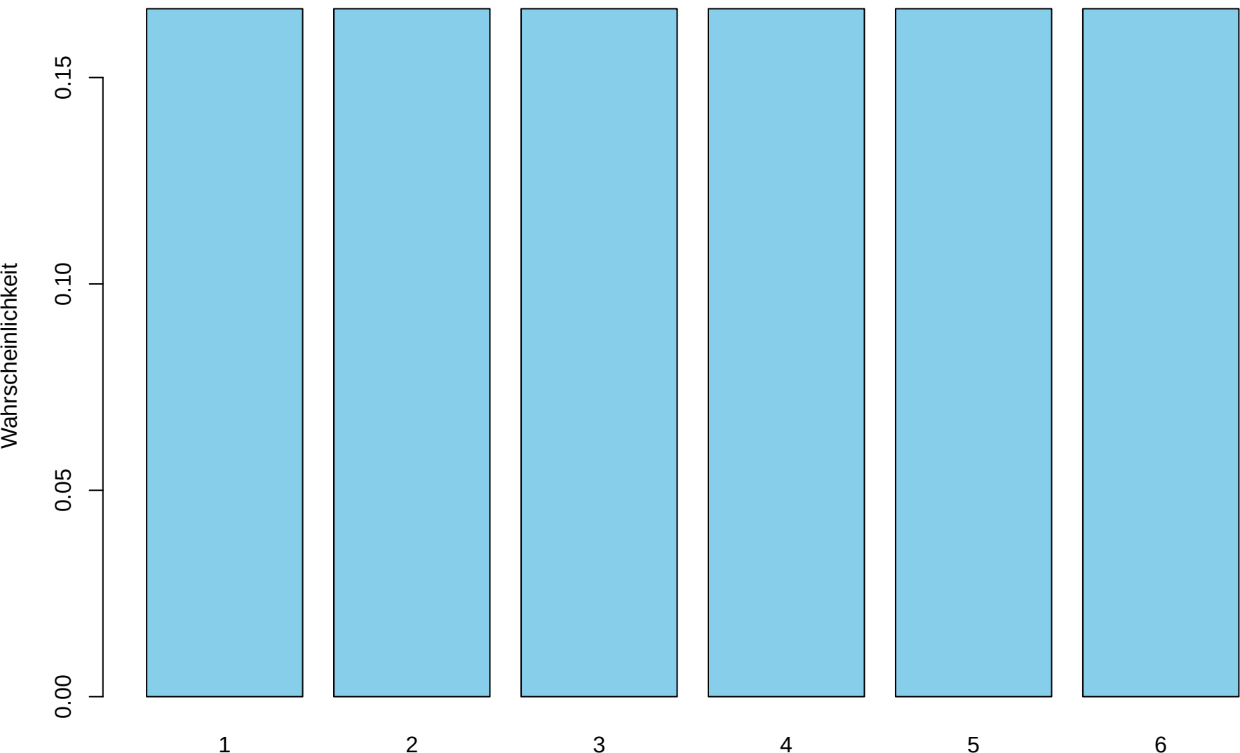
Diskrete Verteilung: Würfelergbeis
