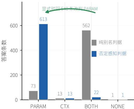
(a) 同一批 649 条答案的判定分配
