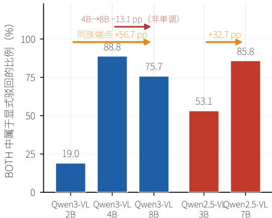
(b) 显式驳回比例随规模上升
