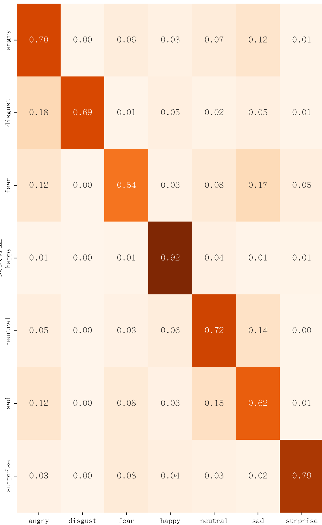
混淆矩阵（归一化）
