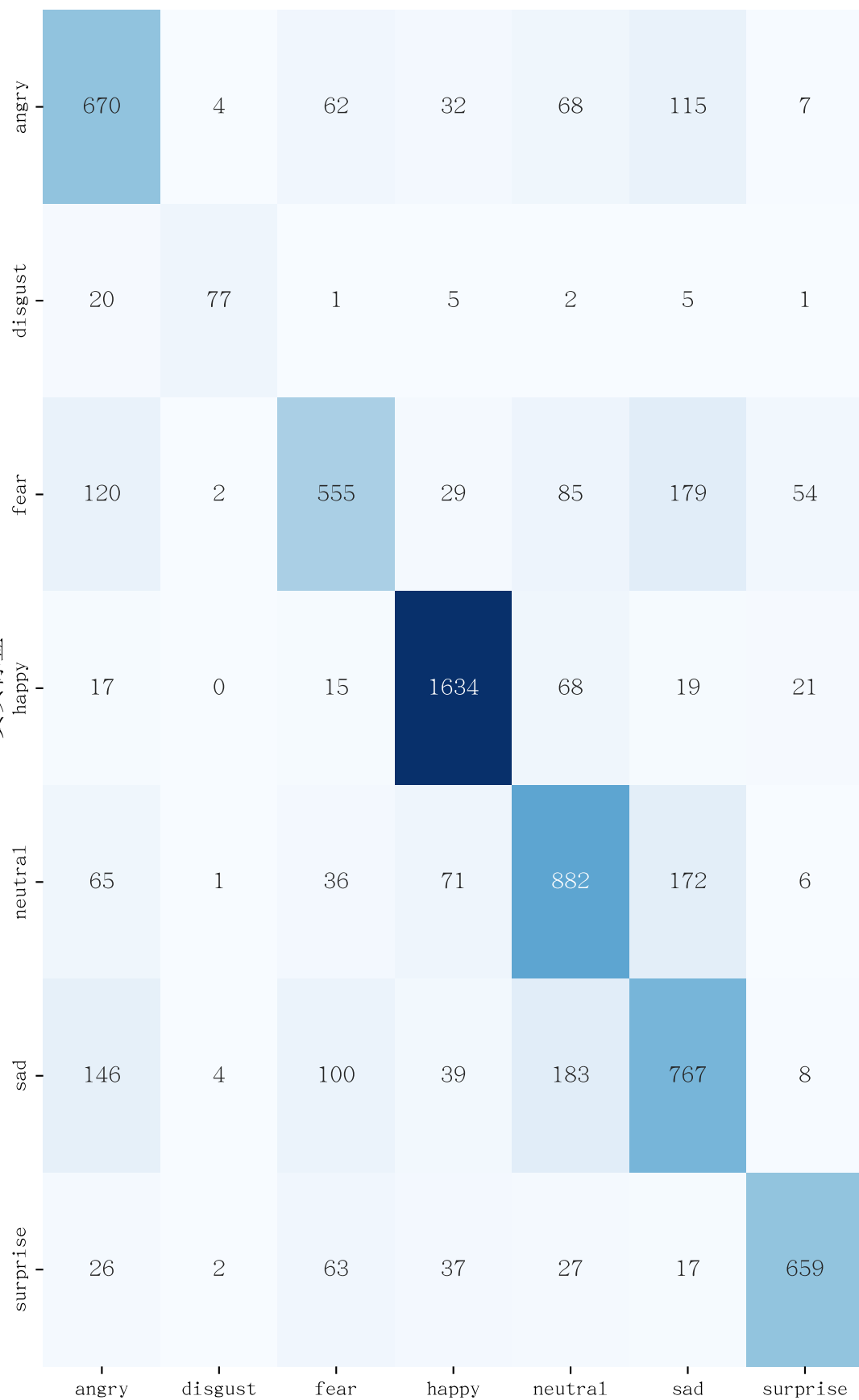
混淆矩阵（原始计数）
