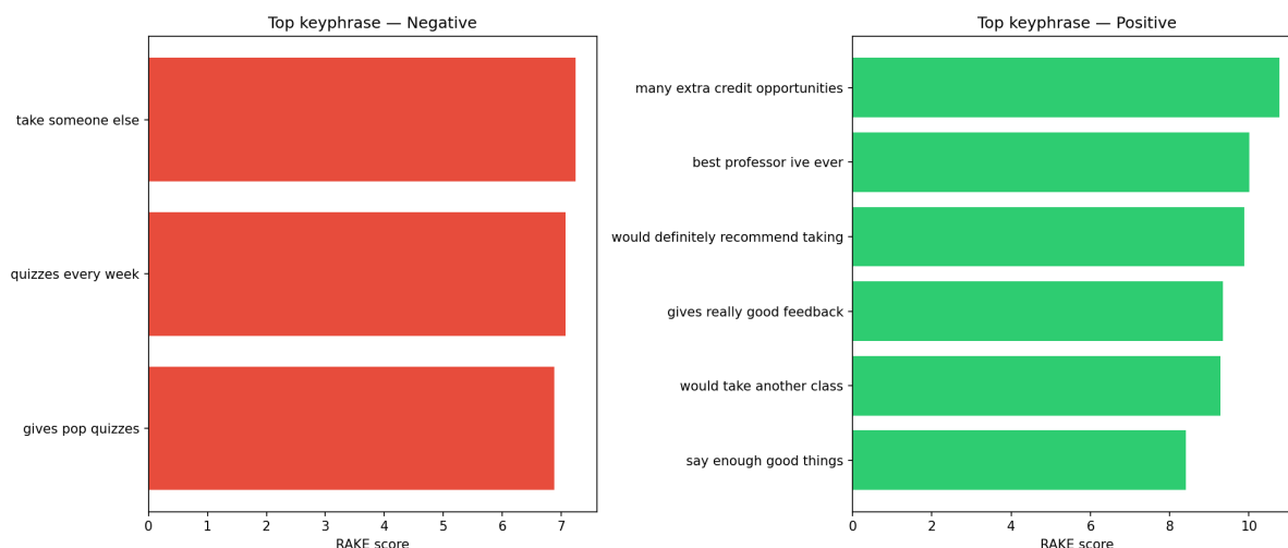
Figura 18: Top keyphrase per classe di sentiment (RAKE)
