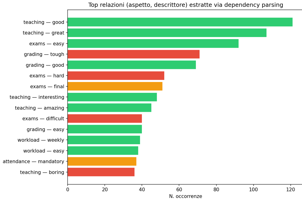
Figura 17: Top relazioni (aspetto, descrittore) estratte via dependency parsing
