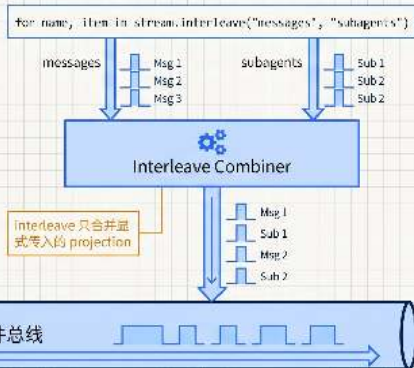
同步程序
