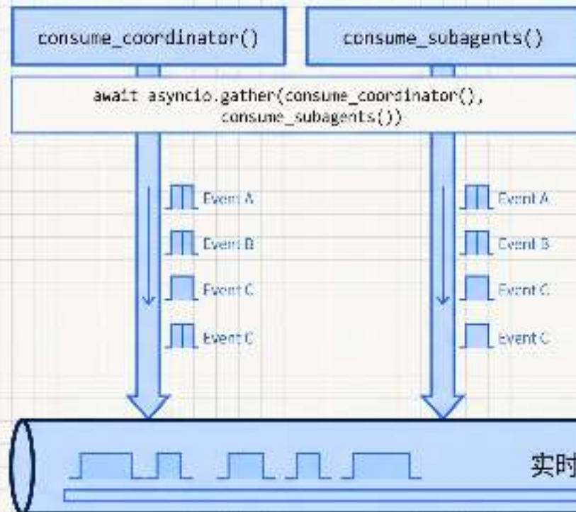
异步服务
