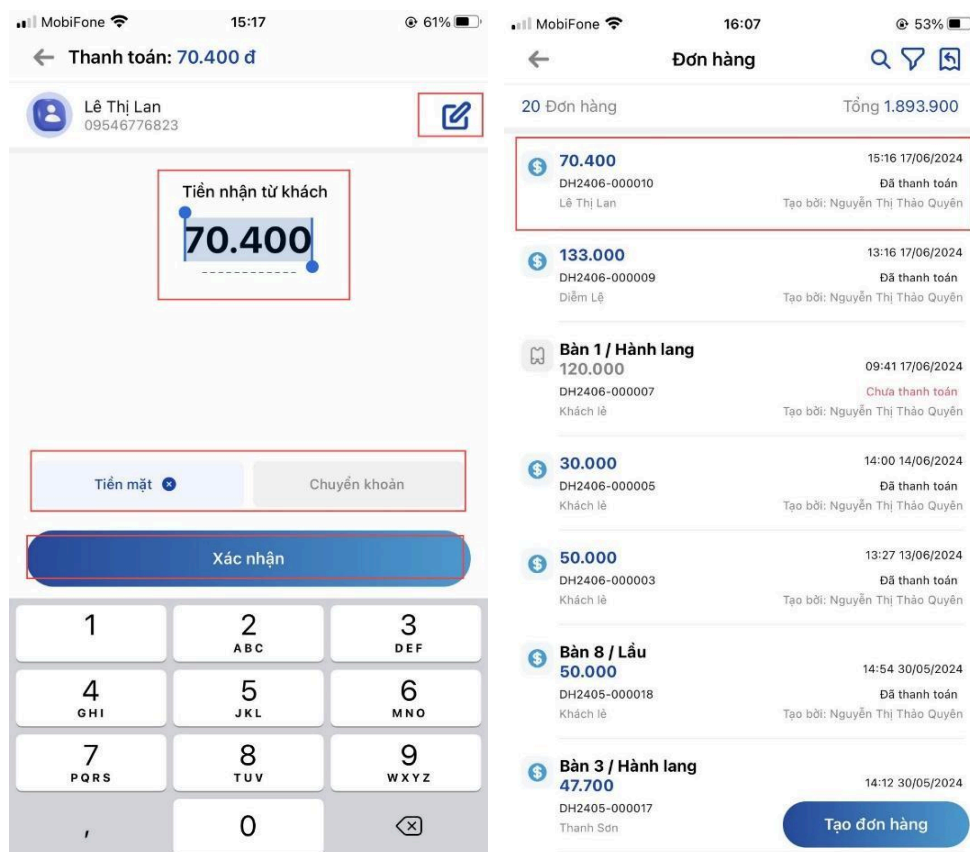
Hình 34: Thanh toán
