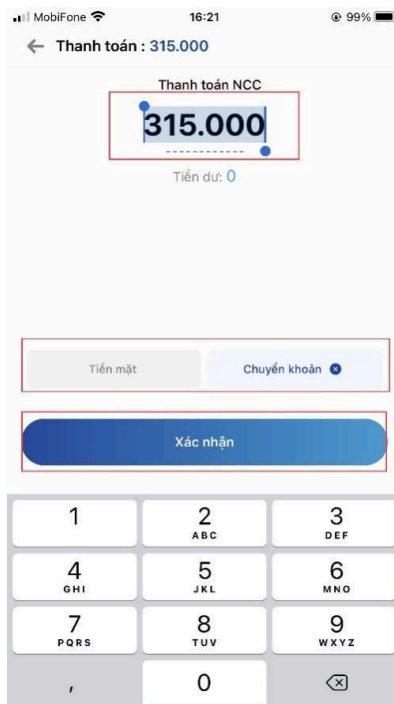
Hình 42: Thanh toán
