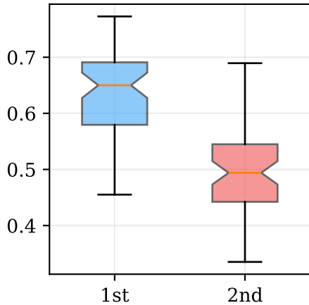
Density (***)
