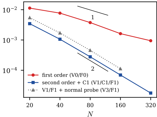
convection--diffusion, Dirichlet
