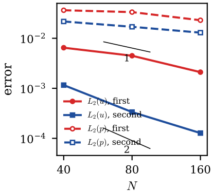
(a) Taylor--Couette
