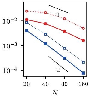
convection--diffusion, Dirichlet
