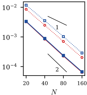
convection--diffusion, Neumann
