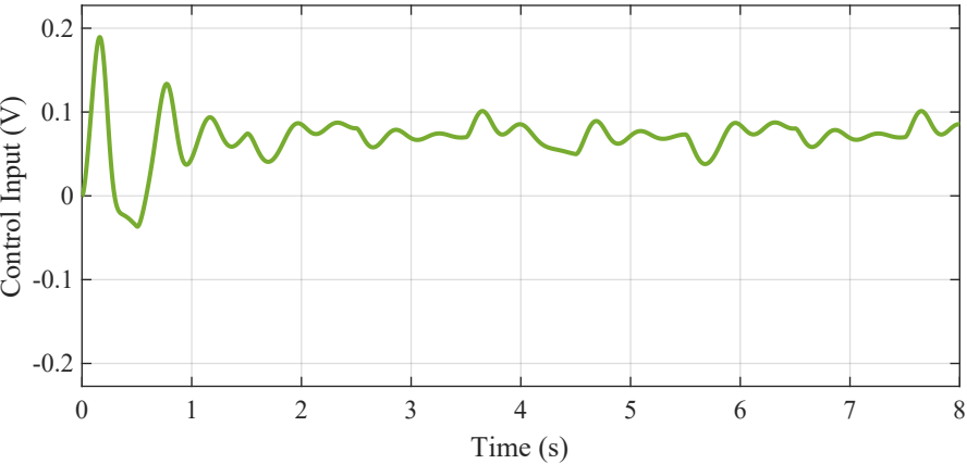
Controller Output Voltage (Pure PID)
