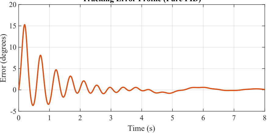
Tracking Error Profile (Pure PID)
