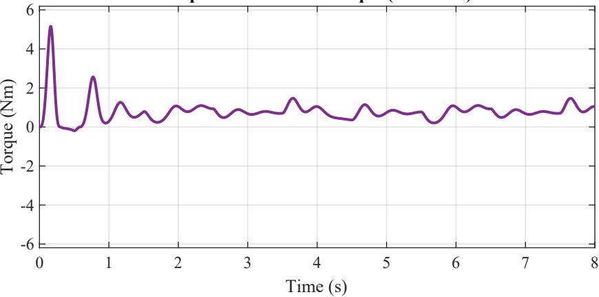
Propeller Generated Torque (Pure PID)
