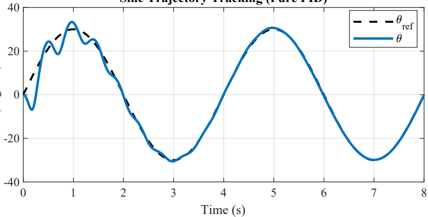
Sine Trajectory Tracking (Pure PID)
