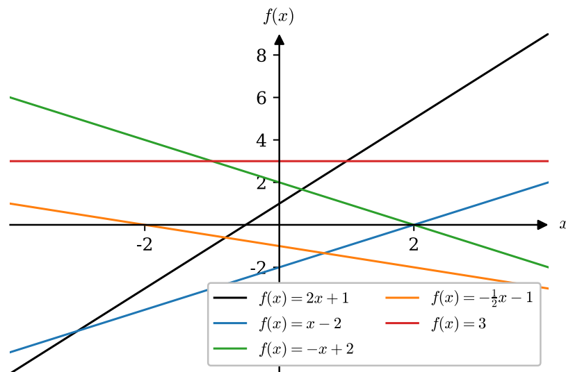
Abbildung 4.22: Fünf affin lineare Funktionen mit unterschiedlicher Steigung und y -Achsenabschnitt.
