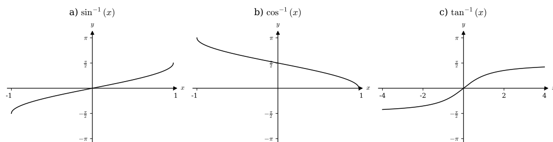
Abbildung 4.44: Arkussinus, Arkuskosinus und Arkustangens.
