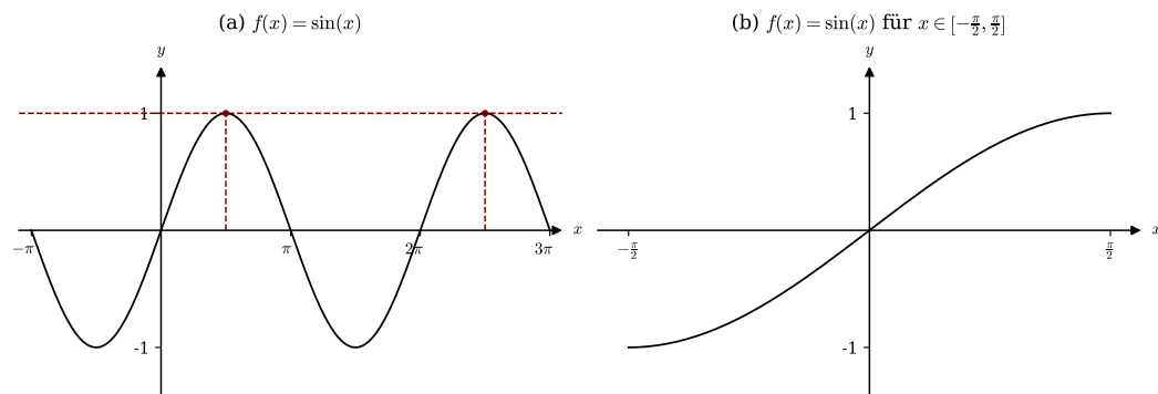
Abbildung 4.18: Graph der Funktion f(x) = \sin(x) . f ist auf ganz \mathbb{R} nicht injektiv (a), auf I = [-\frac{\pi}{2}, \frac{\pi}{2}] jedoch schon (b).
