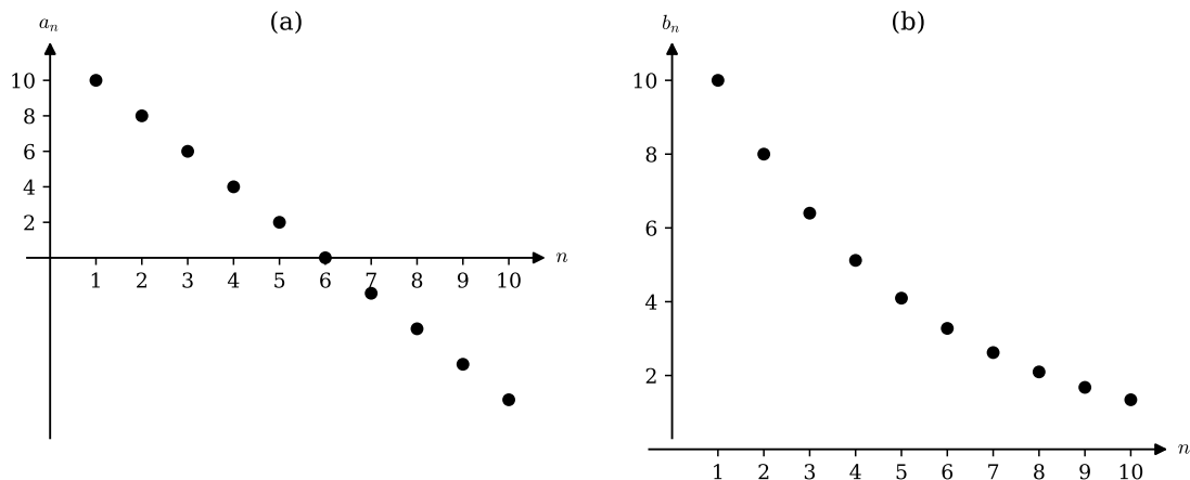
Abbildung 2.5: Arithmetische Folge mit d = -2 (a) und geometrische Folge mit q = 0,8 (b).
