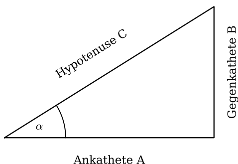
Abbildung 4.34: Rechtwinkliges Dreieck mit Hypotenuse C , Ankathete A und Gegenkathete B .
