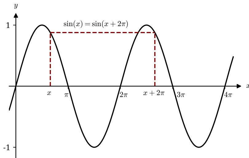
Abbildung 4.12: Die Funktion f(x) = \sin(x) als Beispiel einer periodischen Funktion.
