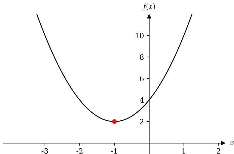
Abbildung 4.24: Parabel f(x) = 2(x + 1)^2 + 2 in Scheitelpunktform. Der Scheitel S = (-1, 2) ist rot markiert.
