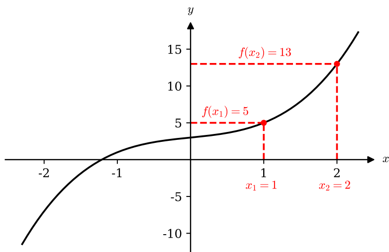
Abbildung 4.6: Monotonieeigenschaften von f(x) = x^3 + x + 3 .
