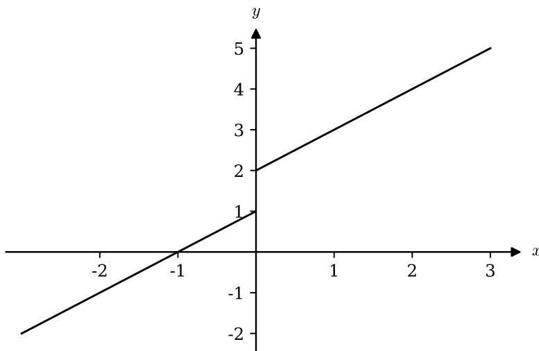
Abbildung 4.14: Graph der stückweise definierten Funktion aus Gleichung 4.9 .
