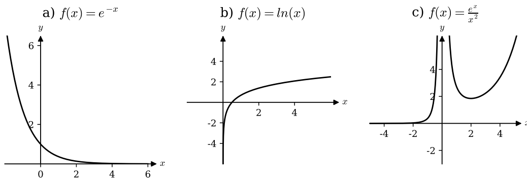
Abbildung 4.7: Beispiele von Funktionen mit verschiedenen Monotonieeigenschaften.
