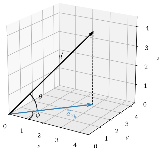
Abbildung 5.14: Richtungswinkel im \mathbb{R}^3 : \phi liegt in der xy -Ebene zwischen der x -Achse und \vec{a}_{xy} , \theta liegt in der von \vec{a}_{xy} und \vec{a} aufgespannten Ebene.
