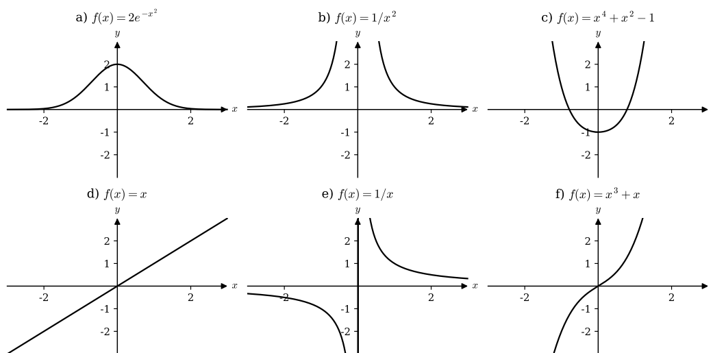
Abbildung 4.11: Weitere Beispiele gerader (a,b,c) und ungerader (d,e,f) Funktionen.
