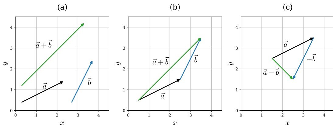
Abbildung 5.7: Veranschaulichung der Vektoraddition.
