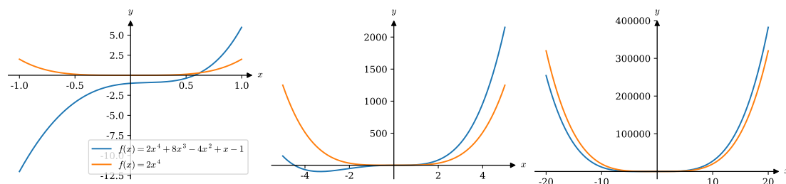
Abbildung 4.26: Verhalten eines Polynoms für große Werte von |x| . Der Wert des Polynoms wird relativ gesehen immer weniger vom höchsten Glied unterscheidbar.
