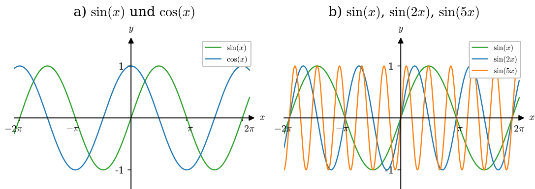
Abbildungung 4.37: Sinus und Kosinus (a) sowie \sin(kx) für verschiedene k (b).
