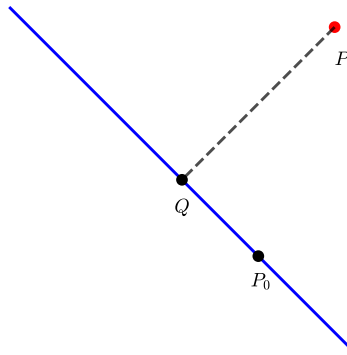
Abbildung 5.21: Abstand eines Punkts zu einer Geraden.
