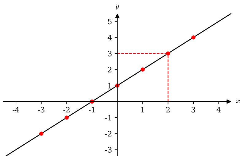
Abbildung 4.2: Graph der Funktion f(x) = x + 1 mit den Werten aus Tabelle 4.1 .
