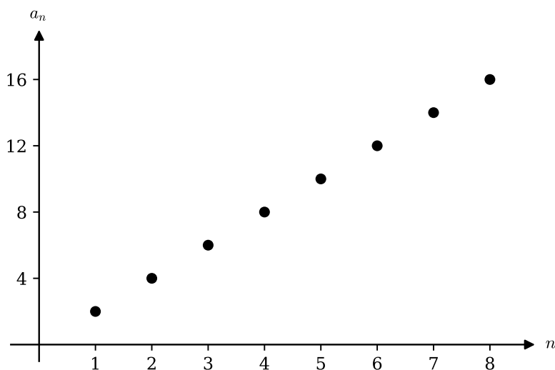
Abbildung 2.1: Visualisierung der ersten acht Glieder der Folge a_n = 2n .
