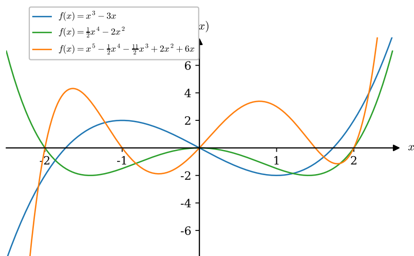
Abbildung 4.25: Beispiele von Polynomen 3., 4. und 5. Grades.
