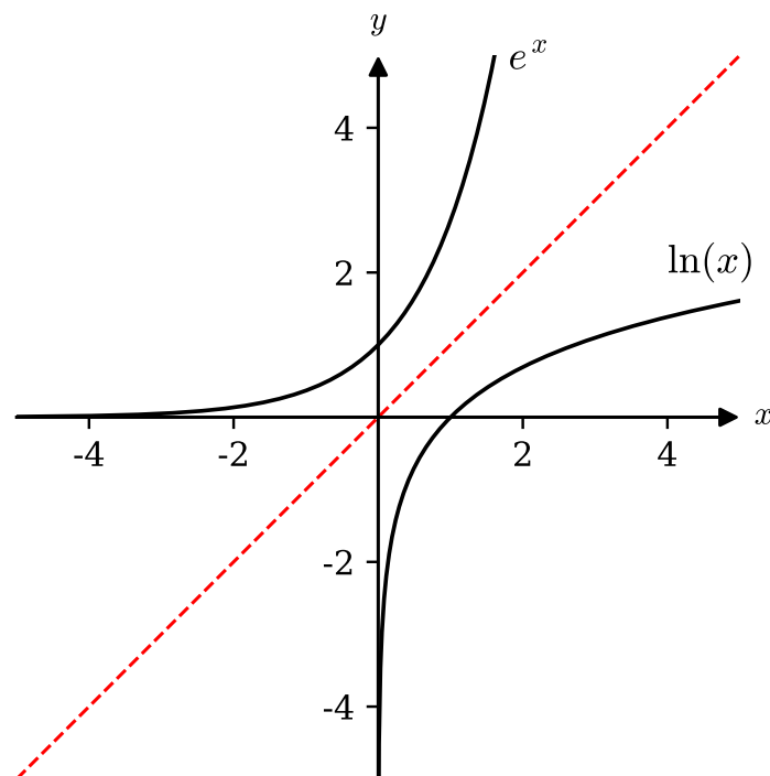
Abbildung 4.20: Die Funktionen f(x) = e^x und f^{-1}(x) = \ln(x) sind zueinander invers. Ihre Graphen entstehen durch Spiegelung an der roten gestrichelten Winkelhalbierenden y = x .
