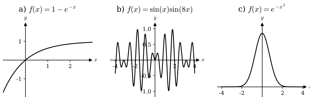
Abbildung 4.8: Beispiele von Funktionen mit verschiedenen Beschränktheitseigenschaften.
