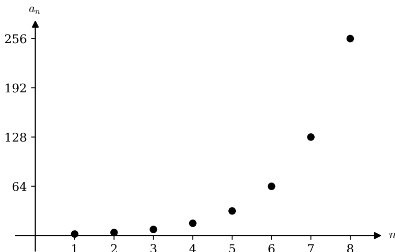
Abbildung 2.2: Visualisierung der ersten acht Glieder der Folge a_n = 2^n .
