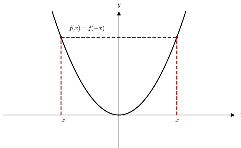
Abbildung 4.9: Zur Definition einer geraden Funktion mit Beispiel einer Parabel f(x) = x^2 .
