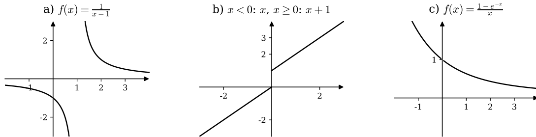
Abbildung 4.16: Beispiele verschiedener Funktionen.
