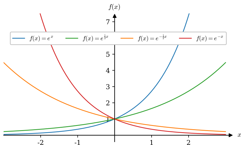
Abbildung 4.29: Beispiele für f(x) = e^{ax} mit positivem und negativem Koeffizienten a .
