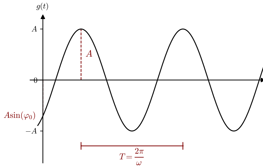
Abbildung 4.43: Harmonische Schwingung.
