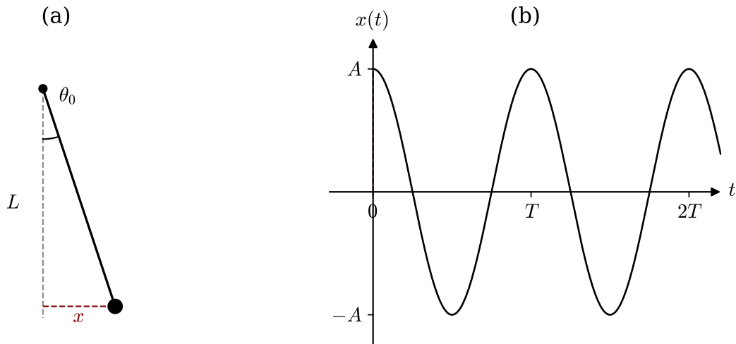
Abbildung 4.44: Mathematisches Pendel: (a) Anfangsauslenkung \theta_0 und x = L \sin(\theta_0) ; (b) x(t) = A \cos(\omega t) mit A = L \sin(\theta_0) .
