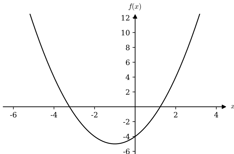
Abbildung 4.5: Graph der Funktion f(x) = x^2 + 2x - 4 .
