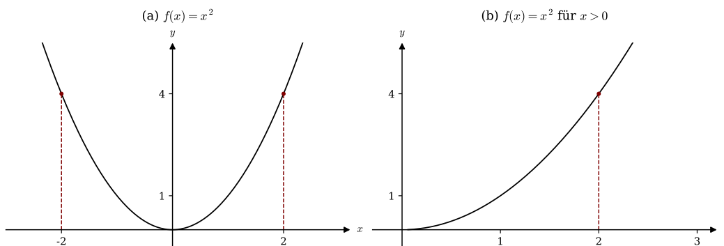
Abbildung 4.19: Der Graph der Funktion f(x) = x^2 . f ist auf ganz \mathbb{R} nicht injektiv (a), auf \mathbb{R}_{>0} jedoch schon (b).
