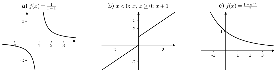
Abbildung 4.18: Beispiele verschiedener Funktionen.
