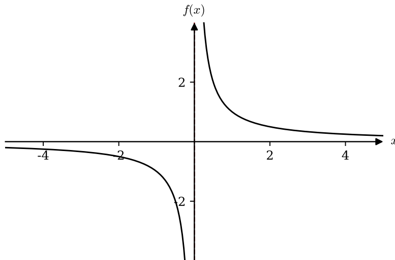
Abbildung 4.17: Graph von f(x) = \frac{1}{x} mit Polstelle bei x = 0 (gestrichelte Linie).
