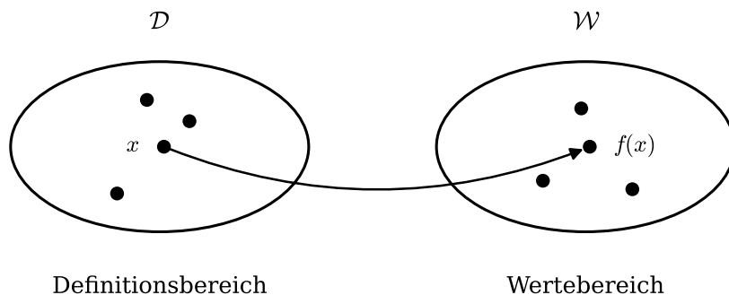
Abbildung 4.1: Schematische Darstellung einer Funktion f als Zuordnung vom Definitionsbereich \mathcal{D} zum Wertebereich \mathcal{W} .
