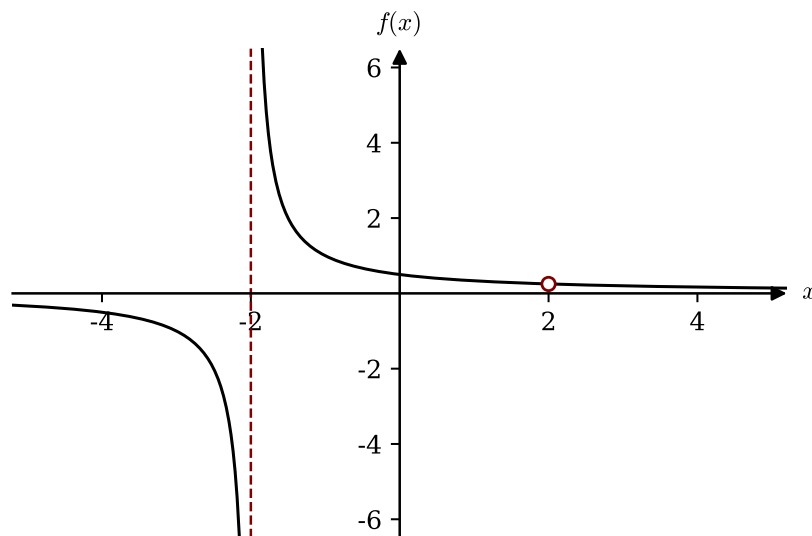
Abbildung 4.34: Die Funktion f(x) = \frac{x-2}{x^2-4} mit Polstelle bei x = -2 und hebbarer Definitionslücke bei x = 2 .
