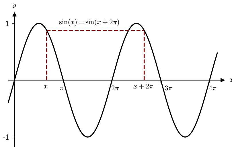
Abbildung 4.13: Die Funktion f(x) = \sin(x) als Beispiel einer periodischen Funktion.
