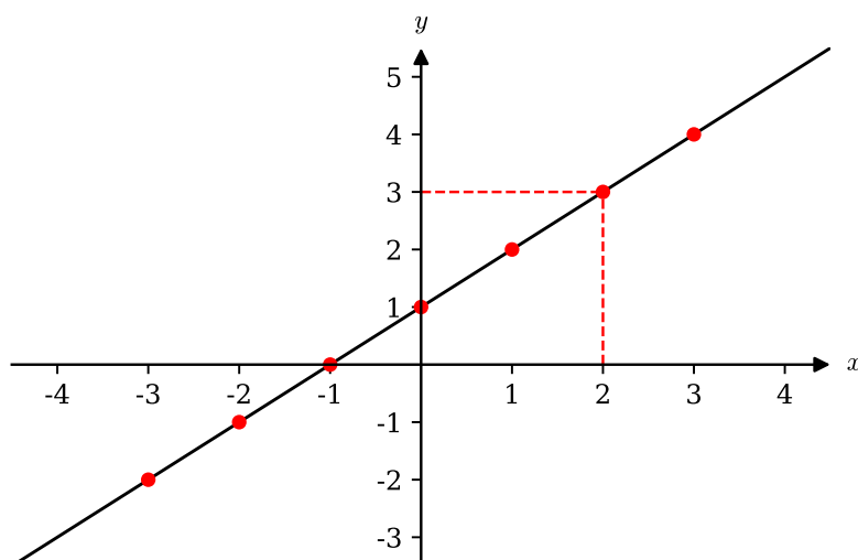
Abbildung 4.2: Graph der Funktion f(x) = x + 1 mit den Werten aus Tabelle 4.1 in rot.
