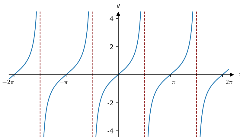
Abbildung 4.40: Die Tangensfunktion mit Polstellen bei x = \frac{\pi}{2} + k\pi (gestrichelte Linien).
