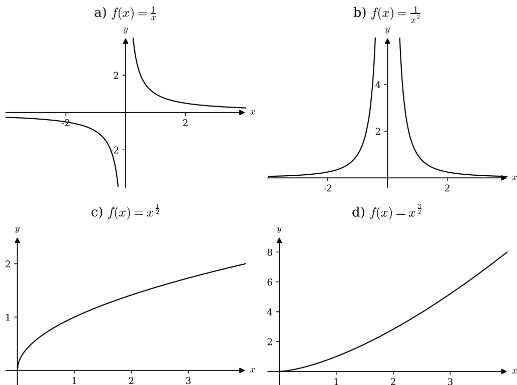
Abbildung 4.29: Beispiele von Potenzfunktionen: Hyperbel \frac{1}{x} , \frac{1}{x^2} , sowie x^{\frac{1}{2}} und x^{\frac{3}{2}} .
