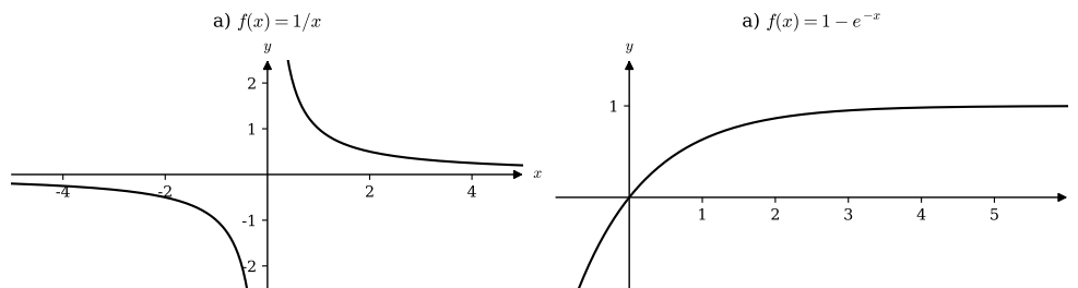
Abbildung 4.16: Beispiele zweier Funktionen mit Konvergenz im Unendlichen.
