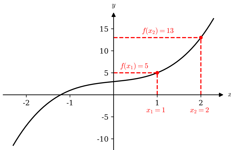
Abbildung 4.7: Monotonieeigenschaften von f(x) = x^3 + x + 3 .
