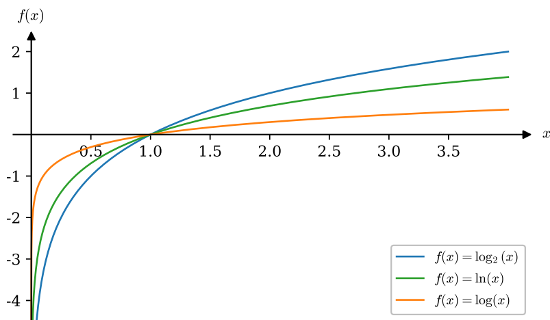
Abbildung 4.32: Logarithmusfunktionen zu den Basen 2, e und 10.
