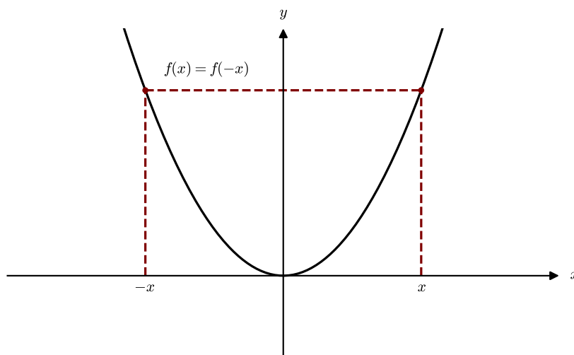
Abbildung 4.10: Zur Definition einer geraden Funktion mit Beispiel einer Parabel f(x) = x^2 .
