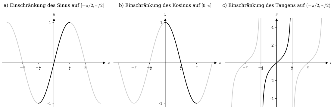
Abbildung 4.45: Injektive Einschränkung von Sinus und Kosinus.
