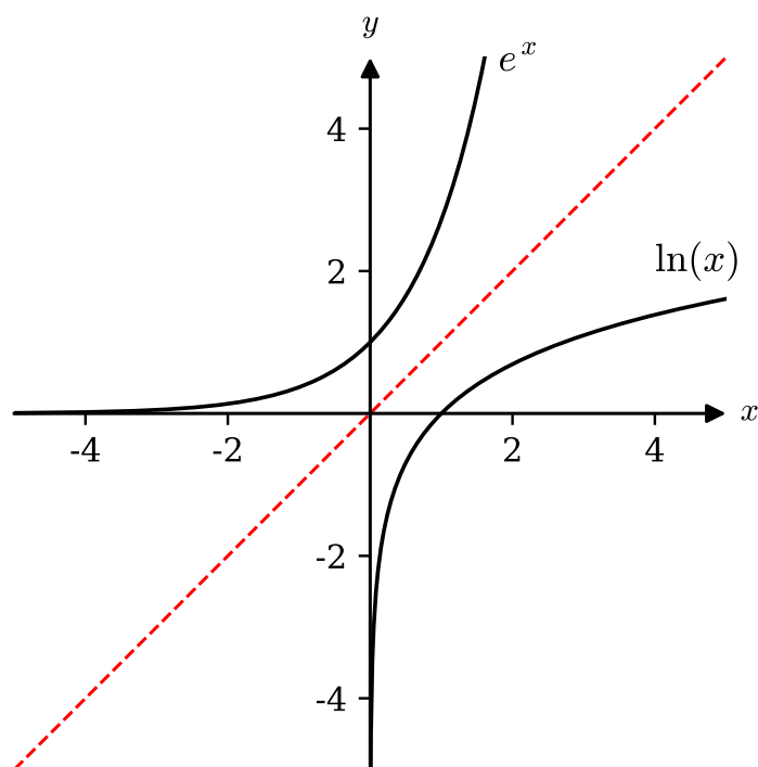
Abbildung 4.22: Die Funktionen f(x) = e^x und f^{-1}(x) = \ln(x) sind zueinander invers. Ihre Graphen entstehen durch Spiegelung an der roten gestrichelten Winkelhalbierenden y = x .
