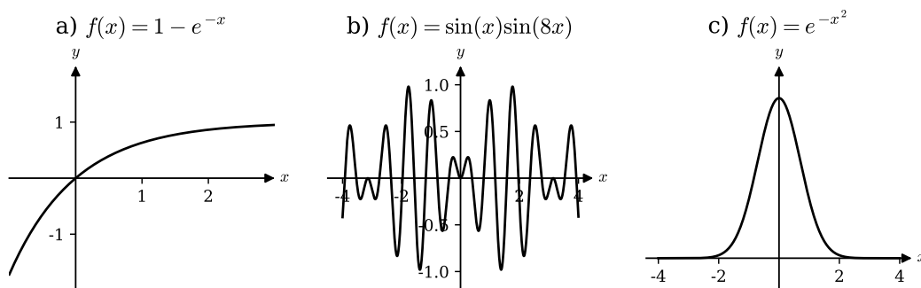
Abbildung 4.9: Beispiele von Funktionen mit verschiedenen Beschränktheitseigenschaften.
