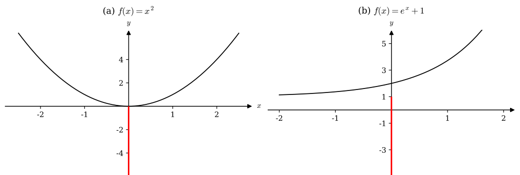
Abbildung 4.21: Surjektivität und Wertebereich zweier Funktionen. Nicht angenommene Werte sind auf der y -Achse rot markiert. Entfernt man diese aus dem Wertebereich, ergeben sich surjektive Funktionen.
