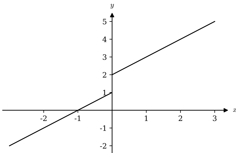
Abbildung 4.15: Graph der stückweise definierten Funktion aus Gleichung 4.9.
