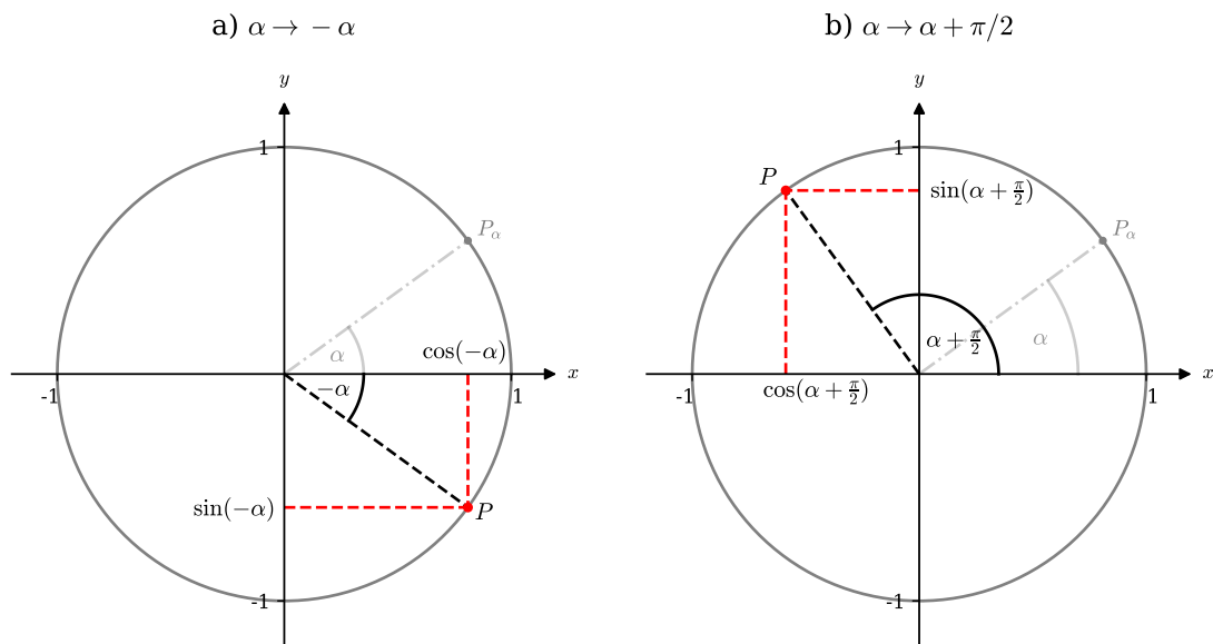
Abbildungung 4.38: Eigenschaften von Sinus und Kosinus unter den Transformationen \alpha \rightarrow -\alpha und \alpha \rightarrow \alpha + \pi/2 .
