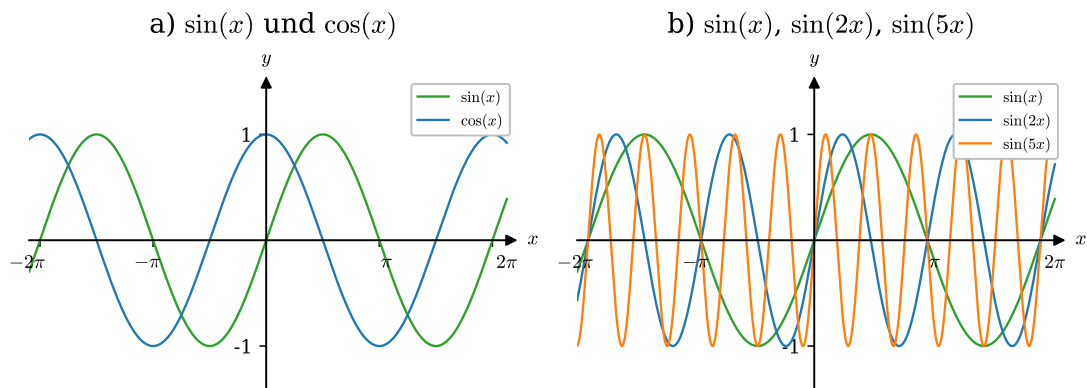
Abbildungung 4.39: Sinus und Kosinus (a) sowie \sin(kx) für verschiedene k (b).
