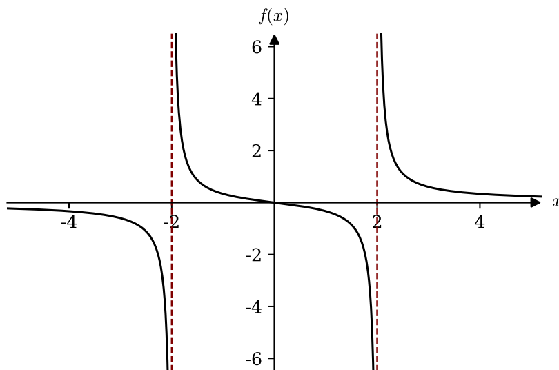
Abbildung 4.33: Die Funktion f(x) = \frac{x}{x^2-4} mit Polstellen bei x = \pm 2 .
