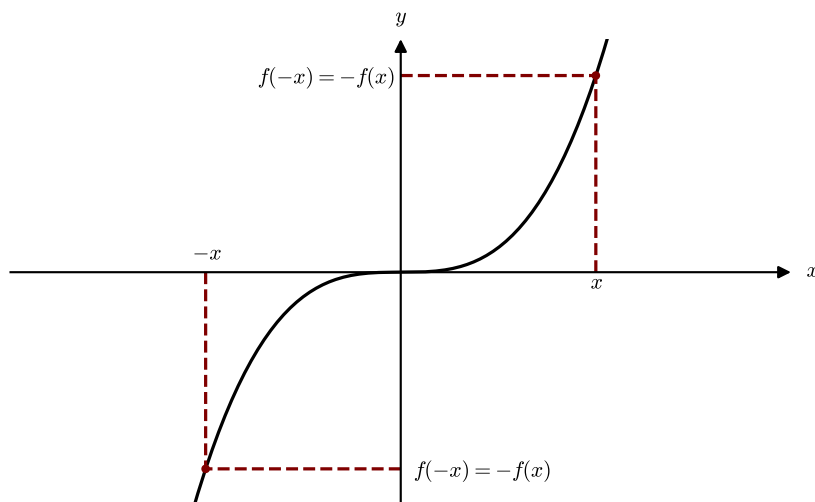
Abbildung 4.11: Zur Definition einer ungeraden Funktion anhand f(x) = x^3 .
