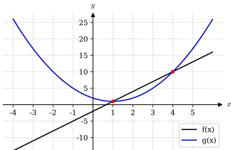
Abbildung 4.6: Funktionsgraphen von f(x) = 3x - 2 und g(x) = x^2 - 2x + 2 , sowie deren Schnittpunkte.
