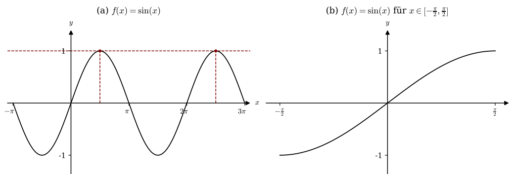
Abbildung 4.20: Graph der Funktion f(x) = \sin(x) . f ist auf ganz \mathbb{R} nicht injektiv (a), auf I = [-\frac{\pi}{2}, \frac{\pi}{2}] jedoch schon (b).
