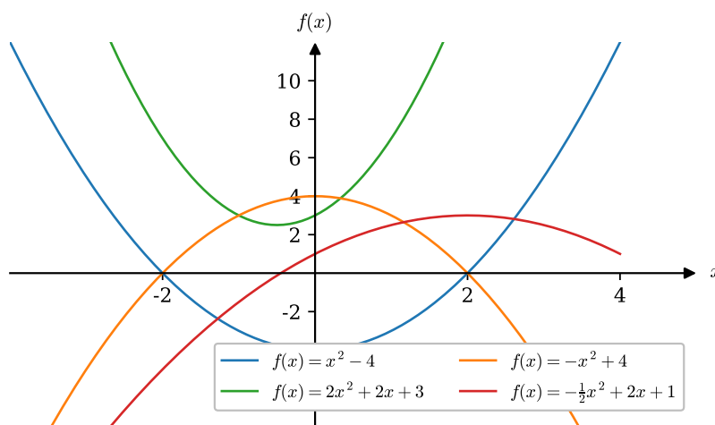
Abbildung 4.25: Beispiele quadratischer Funktionen: zwei Parabeln mit Minimum ( a > 0 ) und zwei mit Maximum ( a < 0 ).
