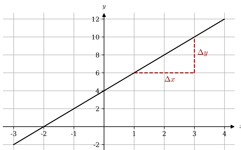
Abbildung 4.23: Graph von f(x) = 2x + 4 mit Steigungsdreieck.
