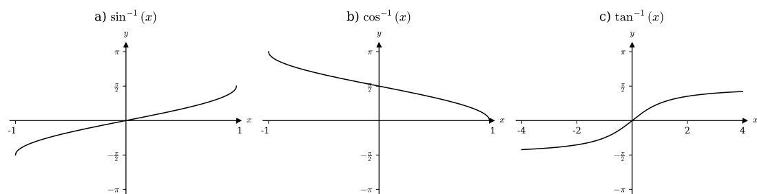
Abbildung 4.44: Arkussinus, Arkuskosinus und Arkustangens.
