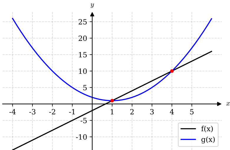
Abbildung 4.5: Funktionsgraphen von f(x) = 3x - 2 und g(x) = x^2 - 2x + 2 , sowie deren Schnittpunkte.
