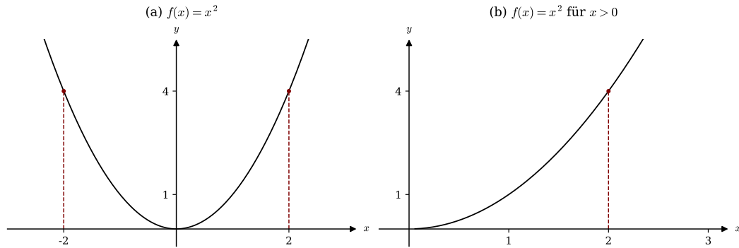
Abbildung 4.17: Der Graph der Funktion f(x) = x^2 . f ist auf ganz \mathbb{R} nicht injektiv (a), auf \mathbb{R}_{\geq 0} jedoch schon (b).
