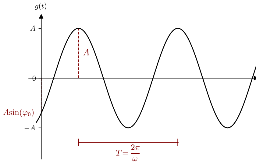
Abbildung 4.41: Harmonische Schwingung.
