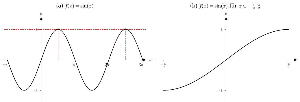
Abbildung 4.17: Graph der Funktion f(x) = \sin(x) . f ist auf ganz \mathbb{R} nicht injektiv (a), auf I = [-\frac{\pi}{2}, \frac{\pi}{2}] jedoch schon (b).
