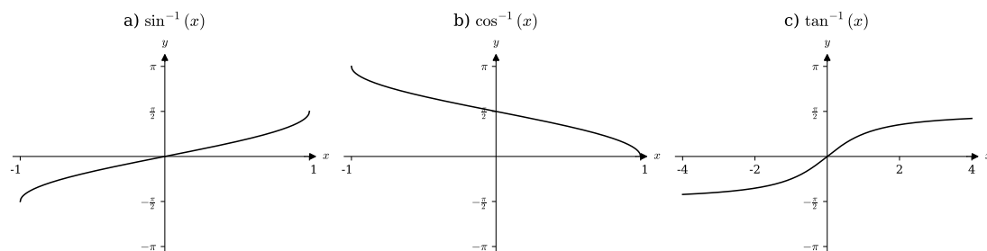
Abbildung 4.41: Arkussinus, Arkuskosinus und Arkustangens.
