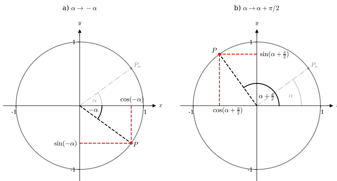
Abbildung 4.35: Eigenschaften von Sinus und Kosinus unter den Transformationen \alpha \rightarrow -\alpha und \alpha \rightarrow \alpha + \pi/2 .
