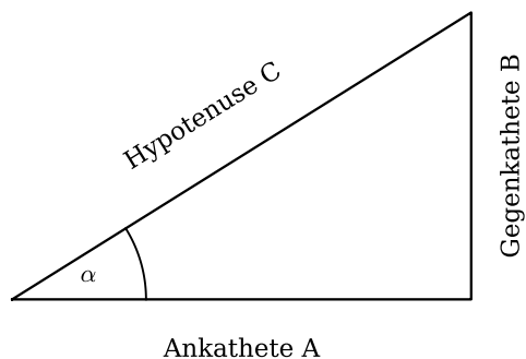
Abbildung 4.33: Rechtwinkliges Dreieck mit Hypotenuse C , Ankathete A und Gegenkathete B .
