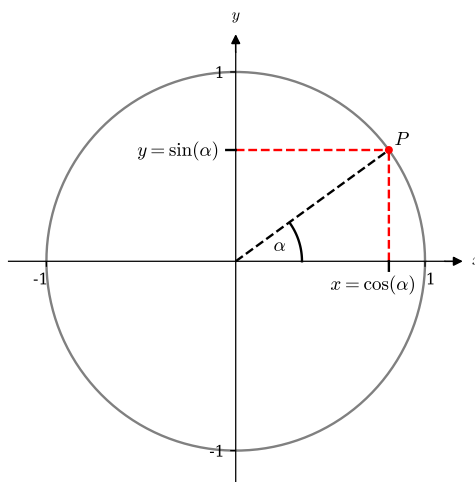
Abbildung 4.34: Definition von Sinus und Kosinus am Einheitskreis.
