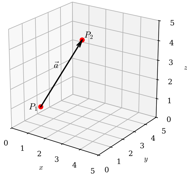
Abbildung 5.13: Vektor \vec{a} von P_1 = (1, 1, 1) nach P_2 = (2, 3, 4) .
