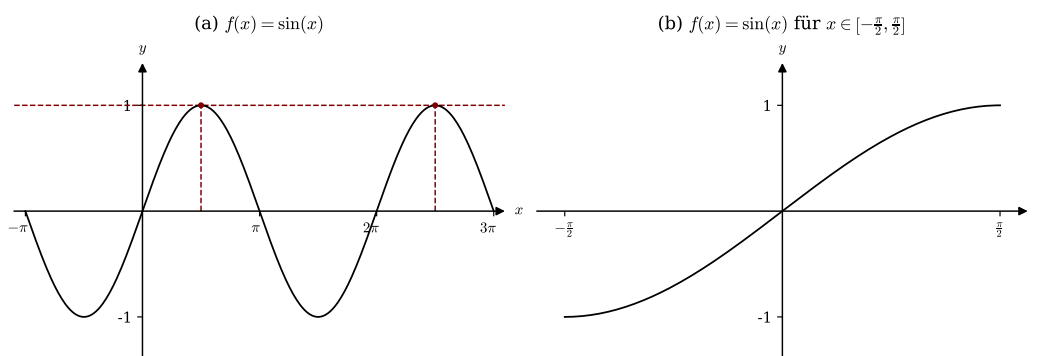
Abbildung 4.18: Graph der Funktion f(x) = \sin(x) . f ist auf ganz \mathbb{R} nicht injektiv (a), auf I = [-\frac{\pi}{2}, \frac{\pi}{2}] jedoch schon (b).
