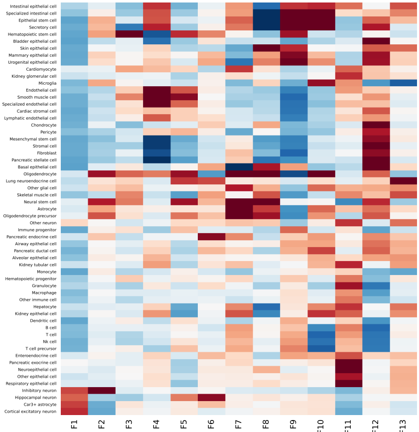
logit homo
