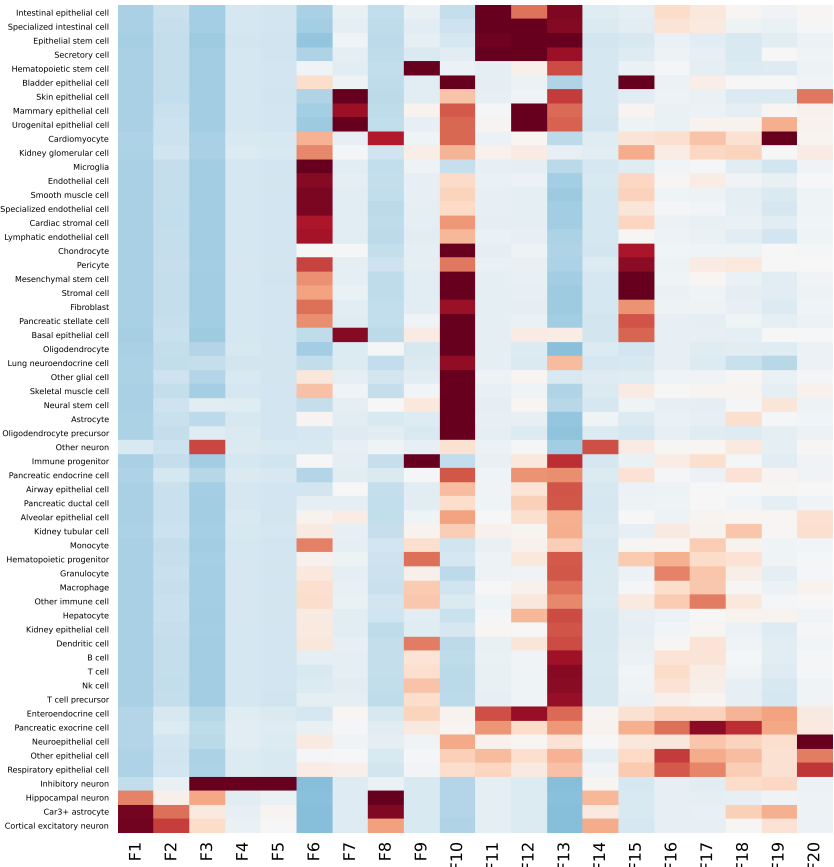
atlas SP
