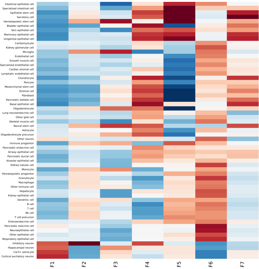
PSI homo
