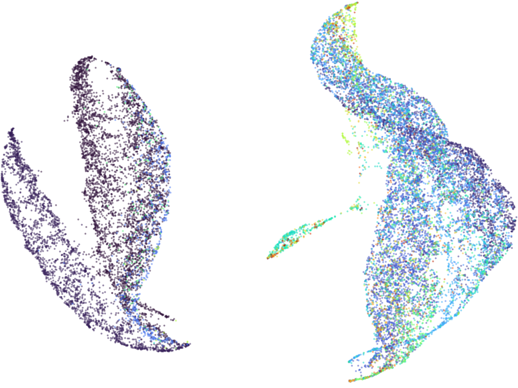
Semi-NMF PSI homo
