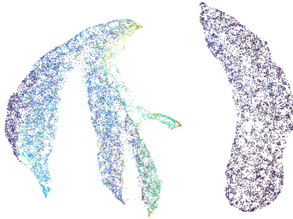
Semi-NMF PSI hetero q25
