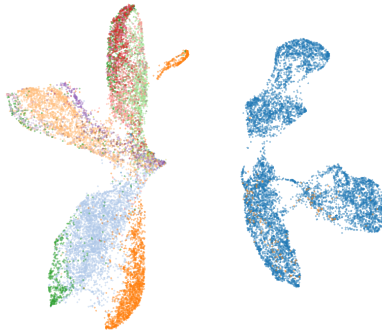
PSI hetero q25
