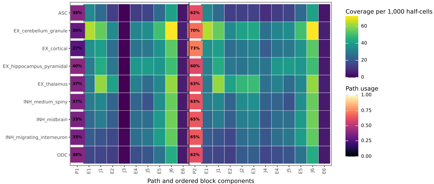
App, poly(dT)
