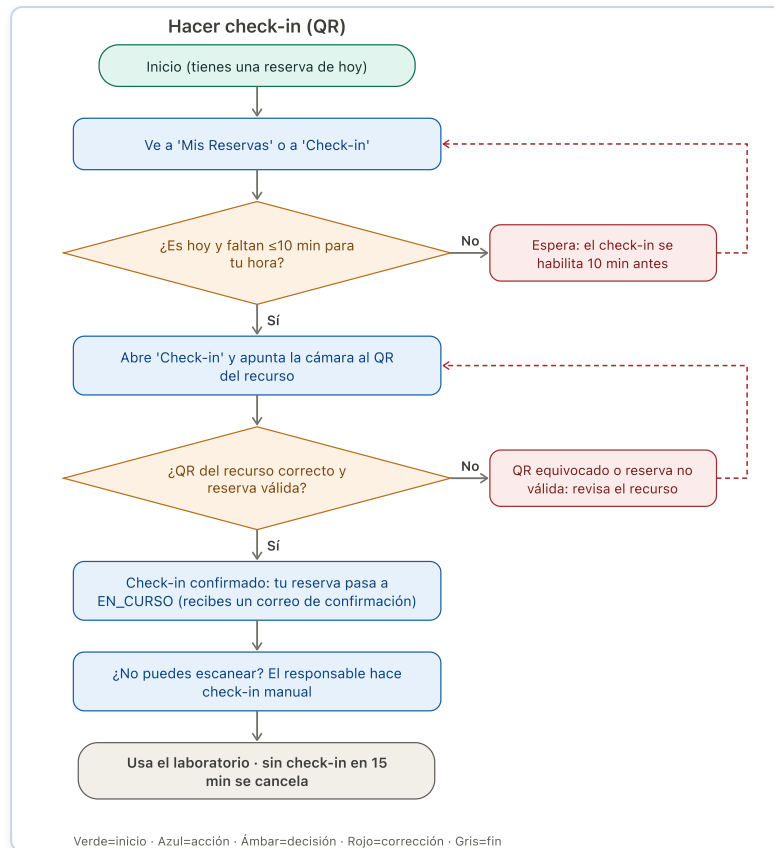
Flujo de check-in.
