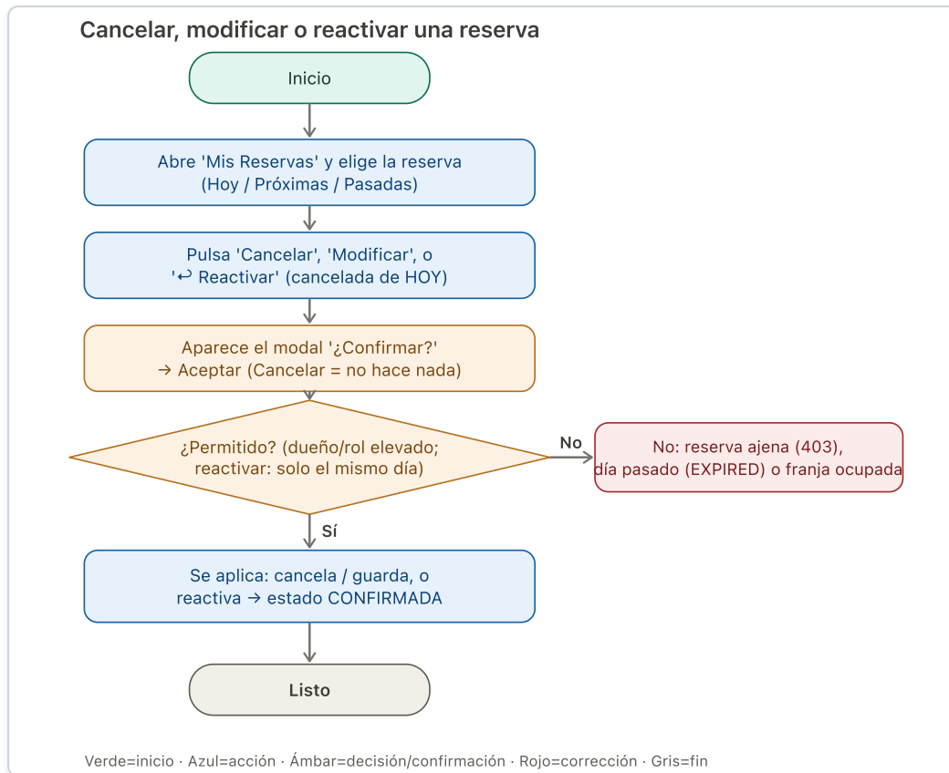
Flujo de cancelación de reserva.
