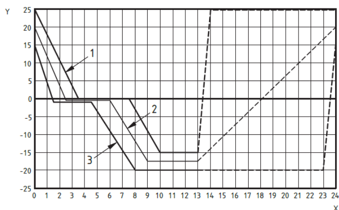
Figura 1. Kurba e temperaturës në qendër të kontenierit të mbushur (pikë matëse referimi) i vendosur në mes të kabinetit
