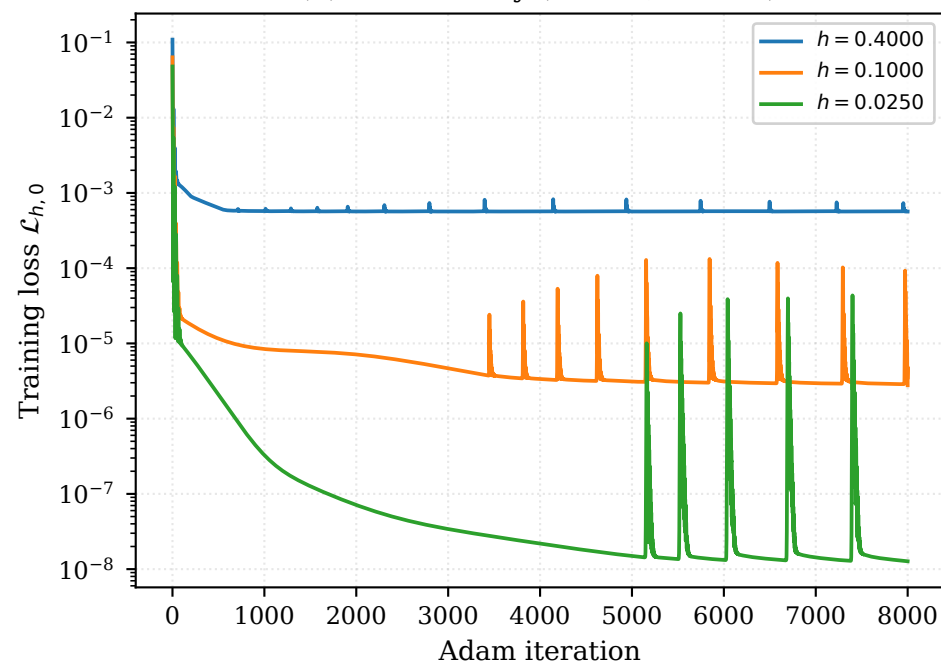
(d) Loss history (seed 0, \alpha = 1.5 )
