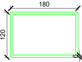
TALPĂ INFERIOARĂ
