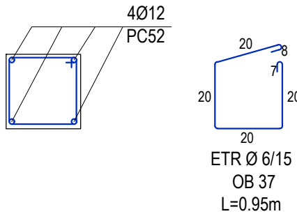
DETALIU STALPISOR S1 25x25 sc 1:25
