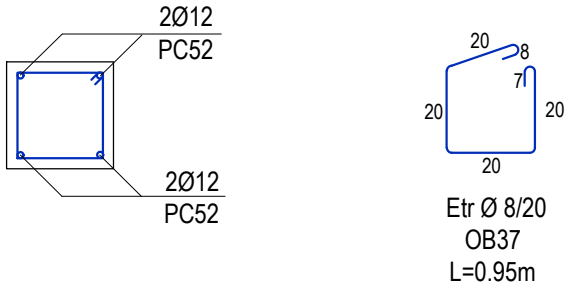
DETALIU ARMARE CENTURA 25x25 sc 1:25
