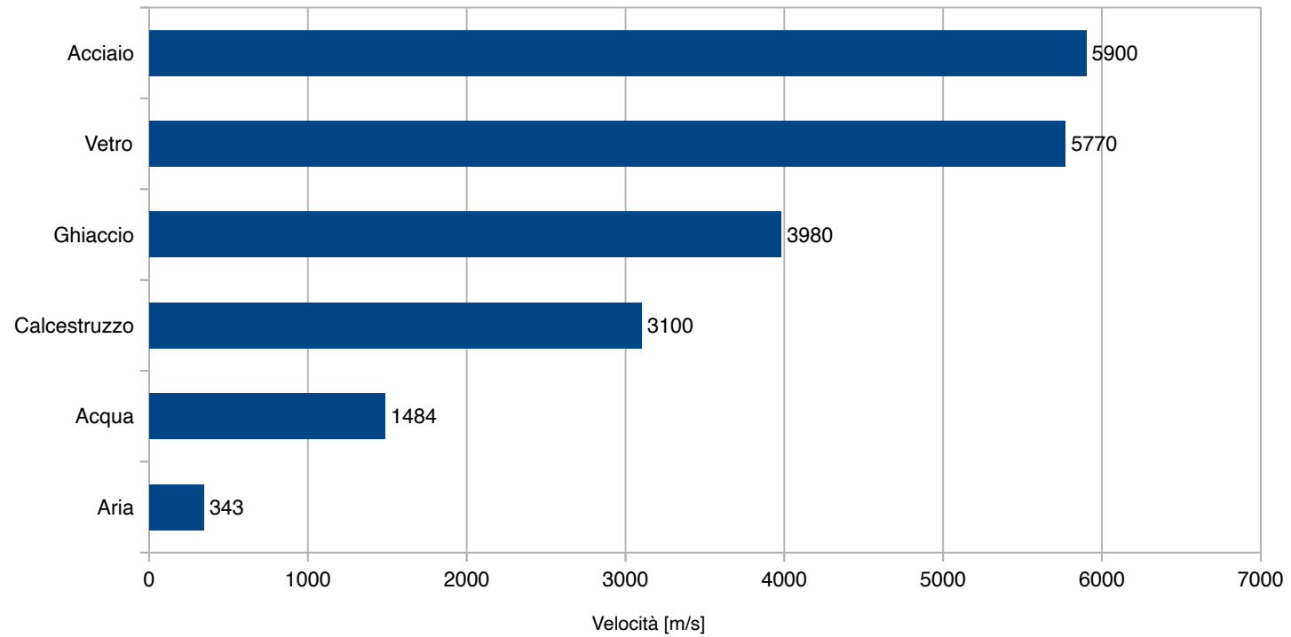
Velocità del suono nei mezzi
