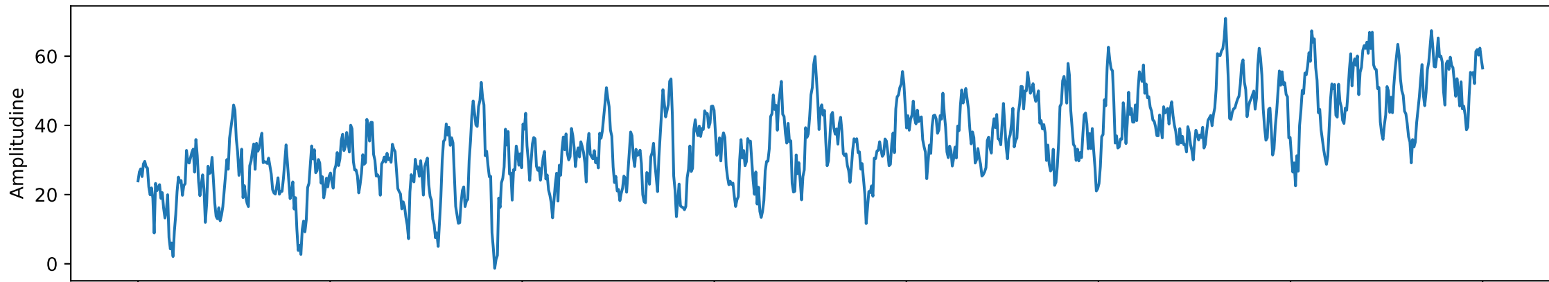
Termeni de eroare epsilon
