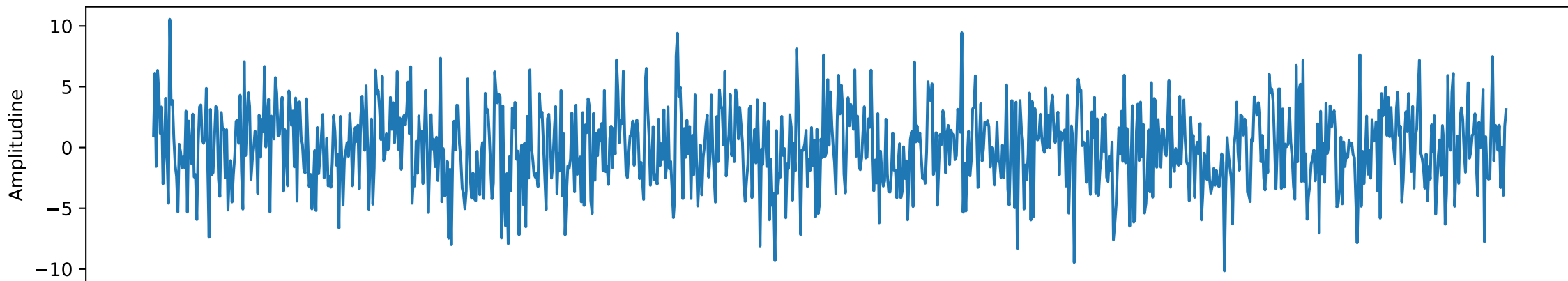
Seria stationara (fara trend si medie)
