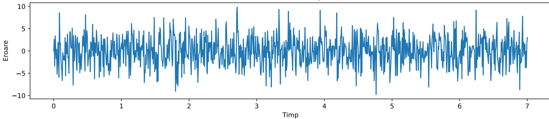
Termeni de eroare epsilon
